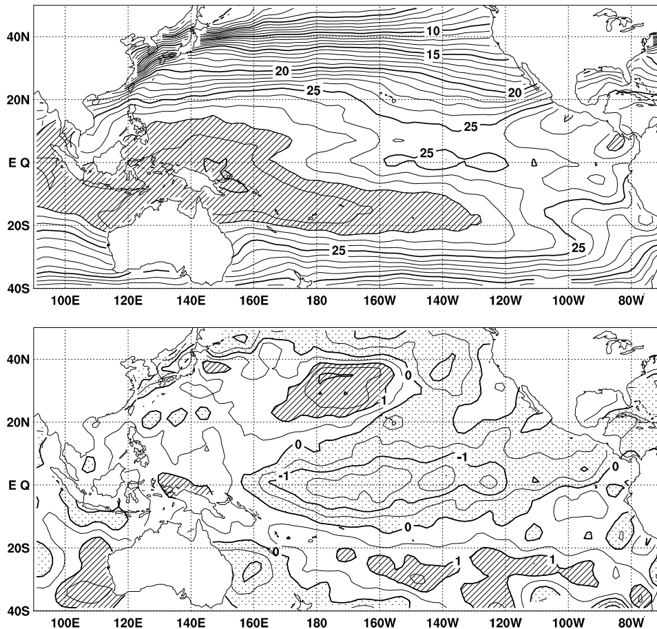
図2 2000年2月の海面水温図(上)及び平年偏差図(下)。海面水温図の太線は5°C毎、細線は1°C毎の、平年偏差図の太線は1°C毎、細線は0.5°C毎の等値線を示す。海面水温図の陰影部は28°C以上の領域を、偏差図の濃い(淡い)陰影部は1°C以上の正偏差域(0°C以下の負偏差域)を示す(平年は1961~90年の30年平均値)。
