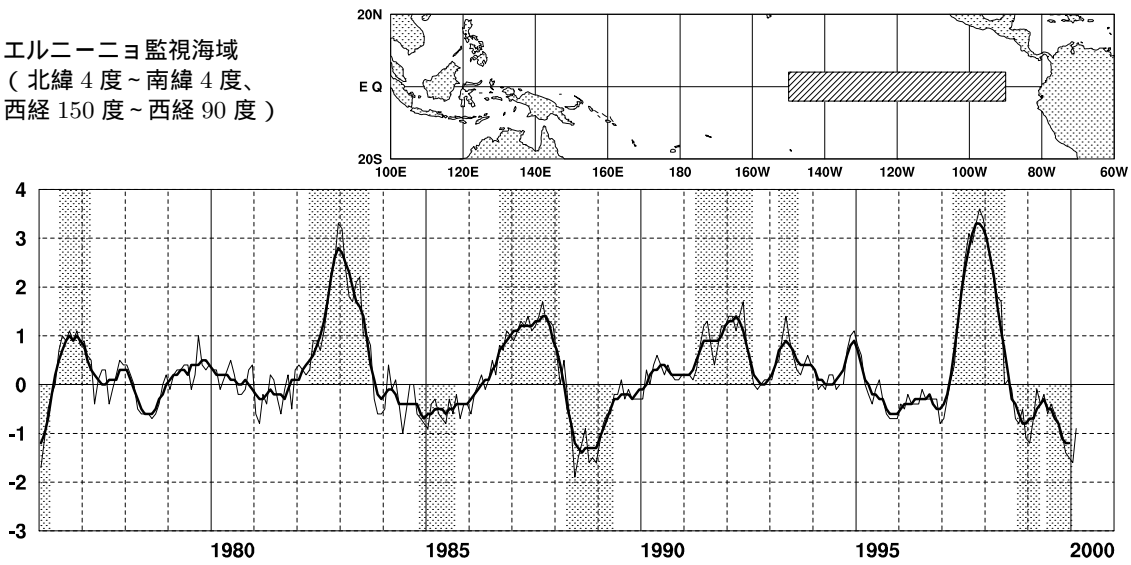
図1 エルニーニョ監視海域の月平均海面水温偏差(°C)の推移(1976年1月~2000年2月)。折線は月平均値、滑らかな太線は5か月移動平均値を示し、正の値は平年(1961~90年の30年平均値)より高いことを示す。エルニーニョ現象の発生期間は上側に、ラニーニャ現象の発生期間は下側に、それぞれ陰影を施してある。
