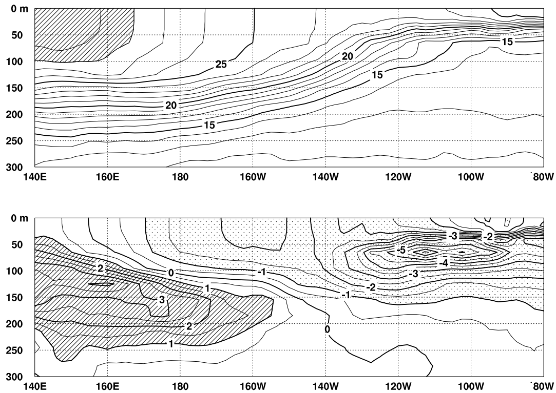
図3 2000年2月の太平洋の赤道に沿った水温(上図)及び平年偏差(下図)の断面図(海洋データ同化システムによる)。上図の等値線間隔は 1^{\circ}\text{C} で 28^{\circ}\text{C} 以上には陰影を施し、下図の等値線間隔は 0.5^{\circ}\text{C} で +1^{\circ}\text{C} 以上( -1^{\circ}\text{C} 以下)の偏差には濃い(薄い)陰影を施した(平年は1987~98年の12年平均値)。
