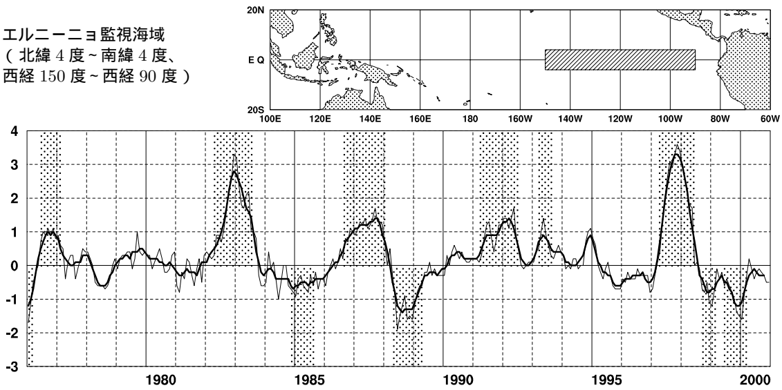
図1 エルニーニョ監視海域の月平均海面水温偏差(°C)の推移(1976年1月~2000年12月)。折線は月平均値、滑らかな太線は5か月移動平均値を示し、正の値は平年(1961~90年の30年平均値)より高いことを示す。エルニーニョ現象の発生期間は上側に、ラニーニャ現象の発生期間は下側に、それぞれ陰影を施してある。
