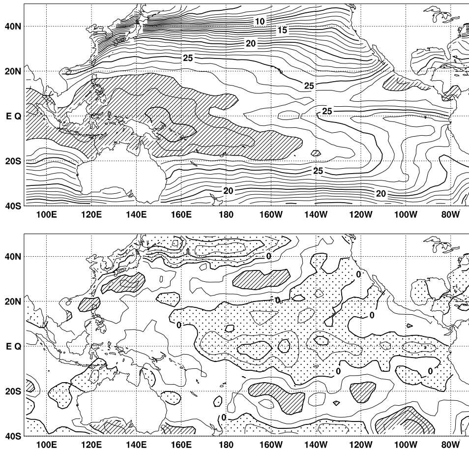
図2 2000年12月の海面水温図(上)及び平年偏差図(下)。海面水温図の太線は5°C毎、細線は1°C毎の、平年偏差図の太線は1°C毎、細線は0.5°C毎の等値線を示す。海面水温図の陰影部は28°C以上の領域を、偏差図の濃い(薄い)陰影部は1°C以上の正偏差域(0°C以下の負偏差域)を示す(平年は1961~90年の30年平均値)。
