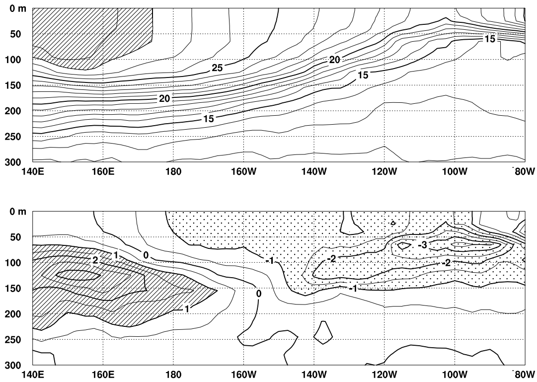
図3 2000年12月の太平洋の赤道に沿った水温(上図)及び年間偏差(下図)の断面図(海洋データ同化システムによる)。上図の等値線間隔は 1^{\circ}\text{C} で 28^{\circ}\text{C} 以上には陰影を施し、下図の等値線間隔は 0.5^{\circ}\text{C} で +1^{\circ}\text{C} 以上( -1^{\circ}\text{C} 以下)の偏差には濃い(薄い)陰影を施した(平年は1987~99年の13年平均値)。
