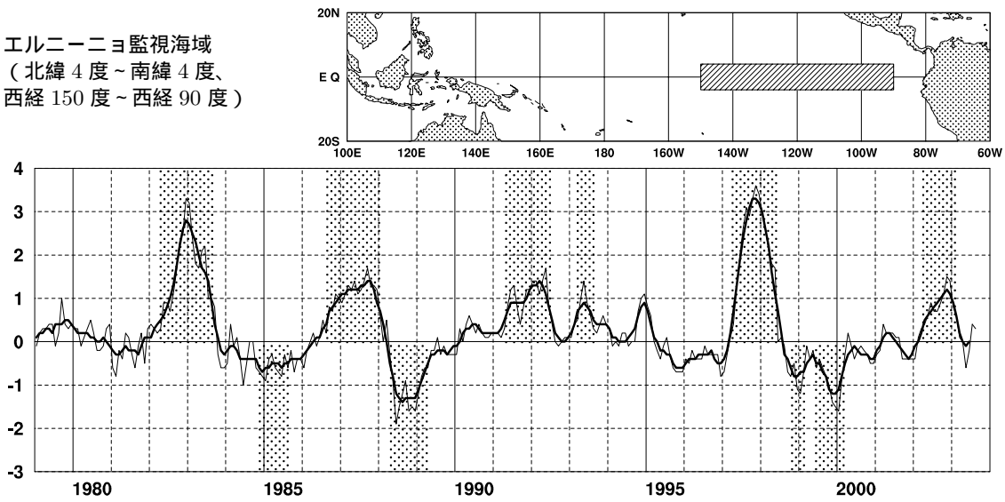
図 1 エルニーニョ監視海域の月平均海面水温の基準値との差 (°C) の推移 (1979 年 1 月 ~ 2003 年 8 月)。折線は月平均値、滑らかな太線は 5 か月移動平均値を示し、正の値は基準値より高いことを示す。エルニーニョ現象の発生期間は上側に、ラニーニャ現象の発生期間は下側に、それぞれ陰影を施してある (基準値は 1961 ~ 1990 年の 30 年平均値)。
