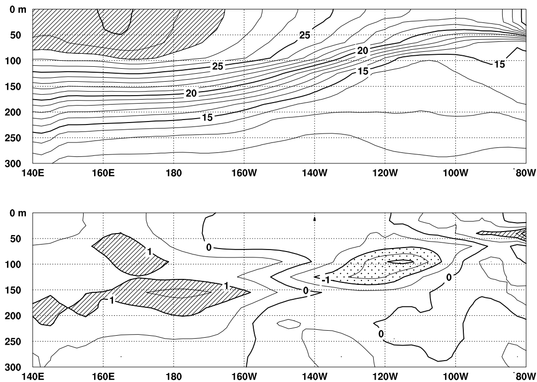
図3 2003年8月の太平洋の赤道に沿った水温(上)及び平年偏差(下)の断面図(海洋データ同化システムによる)。上図の等値線間隔は 1^{\circ}\text{C} で 28^{\circ}\text{C} 以上には陰影を施し、下図の等値線間隔は 0.5^{\circ}\text{C} で +1^{\circ}\text{C} 以上( -1^{\circ}\text{C} 以下)の偏差には濃い(薄い)陰影を施した(平年値は1987~2002年の16年平均値)。
