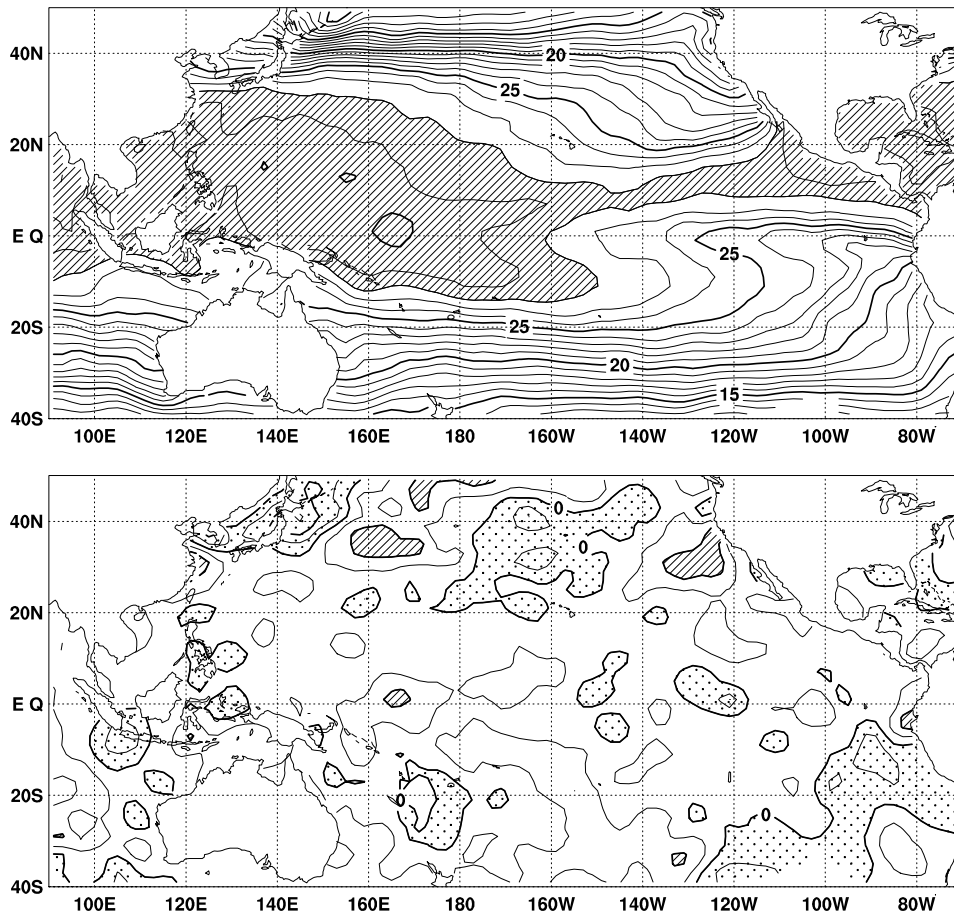
図 2 2003 年 8 月の海面水温図 (上) 及び年偏差図 (下)。海面水温図の大線は 5°C 毎、細線は 1°C 毎の、年偏差図の大線は 1°C 毎、細線は 0.5°C 毎の等値線を示す。海面水温図の陰影部は 28°C 以上の領域を、偏差図の濃い (薄い) 陰影部は +1°C 以上の正偏差域 (0°C 以下の負偏差域) を示す (年偏差は 1971 ~ 2000 年の 30 年平均値)。
