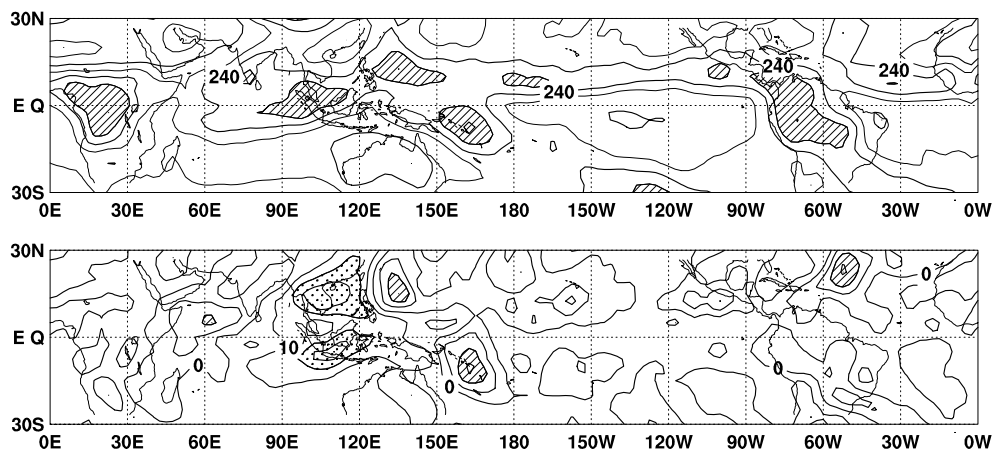
図6 2004年10月の外向き長波放射量(OLR)(上)及び平年偏差(下)の分布図。OLRの値が小さいほど、対流活動が活発であることを示しており、上図では 220\text{W}/\text{m}^2 以下の領域に陰影を、下図ではOLRが平年値より 20\text{W}/\text{m}^2 以上少ない(多い)領域に濃い(薄い)陰影を施した(平年値は1979~2000年の22年平均値)。上図は 20\text{W}/\text{m}^2 毎、下図は 10\text{W}/\text{m}^2 毎に等値線を描いている。OLRデータは米国海洋大気庁(NOAA)から提供されたものである。
