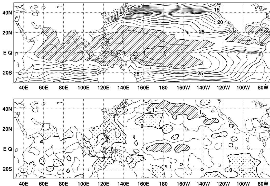
図2 2004年10月の海面水温図(上)及び平年偏差図(下)。海面水温図の太線は 5^{\circ}\text{C} 毎、細線は 1^{\circ}\text{C} 毎の、平年偏差図の太線は 1^{\circ}\text{C} 毎、細線は 0.5^{\circ}\text{C} 毎の等値線を示す。海面水温図の陰影部は 28^{\circ}\text{C} 以上の領域を示し、偏差図の濃い陰影部は海面水温が平年値より 1^{\circ}\text{C} 以上高い領域を、薄い陰影部は平年値より低い領域を示す (平年値は1971~2000年の30年平均値)。
