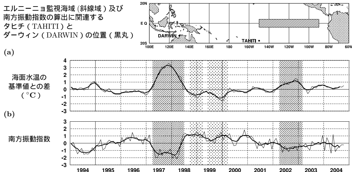
図1 エルニーニョ監視海域の海面水温の基準値との差 ( ^{\circ}\text{C} ) (a) と南方振動指数 (b) の推移 (1994年1月～2004年10月)。折線は月平均値、滑らかな太線は5か月移動平均値を示す（海面水温の基準値は1961～1990年の30年平均値、南方振動指数の年平均値は1971～2000年の30年平均値）。エルニーニョ現象の発生期間に濃い陰影を、ラニーニャ現象の発生期間に淡い陰影を施した。
