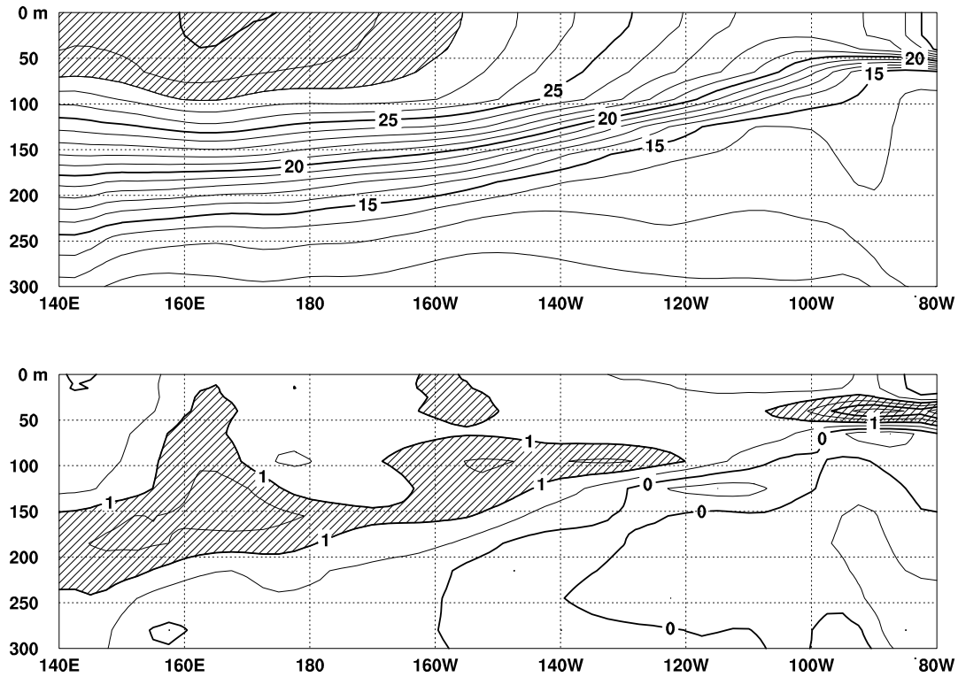
図3 2004年10月の太平洋の赤道に沿った水温(上)及び平年偏差(下)の断面図(海洋データ同化システムによる)。上図の等値線間隔は 1^{\circ}\text{C} で 28^{\circ}\text{C} 以上には陰影を施し、下図の等値線間隔は 0.5^{\circ}\text{C} で、水温が平年値より 1^{\circ}\text{C} 以上高い(低い)領域には濃い(薄い)陰影を施した(平年値は1987~2003年の17年平均値)。
