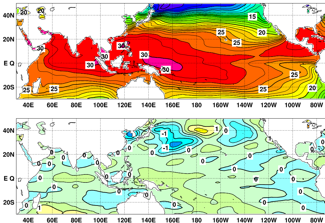
図 2 2006 年 6 月の海面水温図 ( 上 ) 及び平年偏差図 ( 下 )、海面水温図の太線は 5^{\circ}\text{C} 毎、細線は 1^{\circ}\text{C} 毎の、平年偏差図の太線は 1^{\circ}\text{C} 毎、細線は 0.5^{\circ}\text{C} 毎の等値線を示す ( 平年値は 1971 ~ 2000 年の 30 年平均値 )
