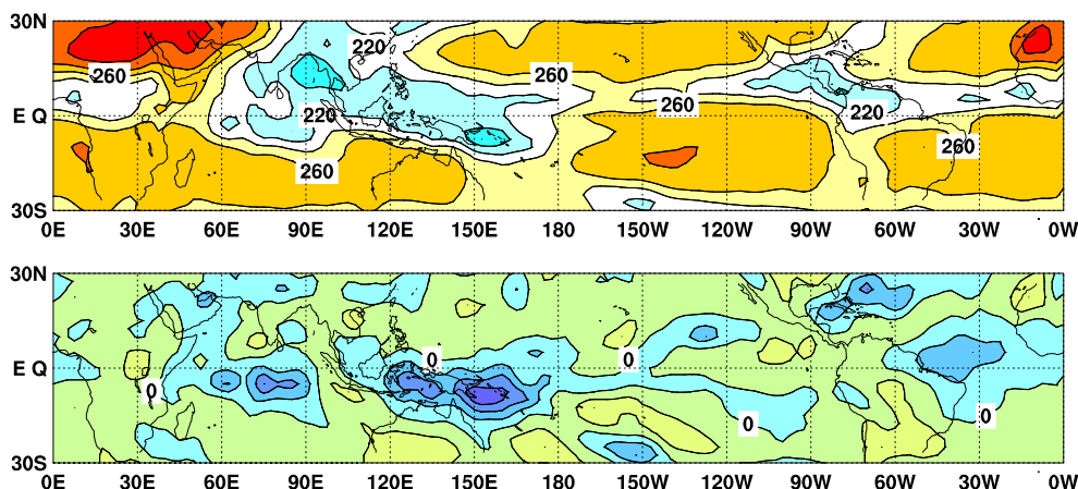
図 6 2006年6月の外向き長波放射量(OLR)(上)及び平年偏差(下)の分布図。OLRの値が小さいほど、対流活動が活発であることを示す。上図は 20\text{W}/\text{m}^2 毎、下図は 10\text{W}/\text{m}^2 毎に等値線を描いている(平年値は1979~2000年の22年平均値)。OLRデータは米国海洋大気庁(NOAA)から提供されたものである。
