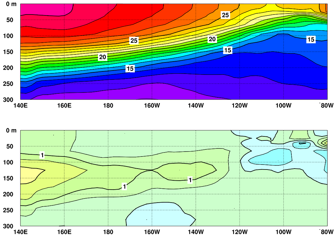
図3 2006年6月の太平洋の赤道に沿った水温(上)及び年間偏差(下)の断面図(海洋データ同化システムによる)。上図の等値線間隔は 1^{\circ}\text{C} 、下図の等値線間隔は 0.5^{\circ}\text{C} (年平均値は1987~2005年の19年平均値)。
