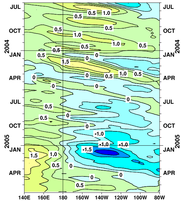
図5 太平洋の赤道に沿った海面から深度260mまでの平均水温年間偏差の経度-時間断面図(海洋データ同化システムによる)。等値線の間隔は 0.5^{\circ}\text{C} (年平均値は1987~2005年の19年平均値)。
