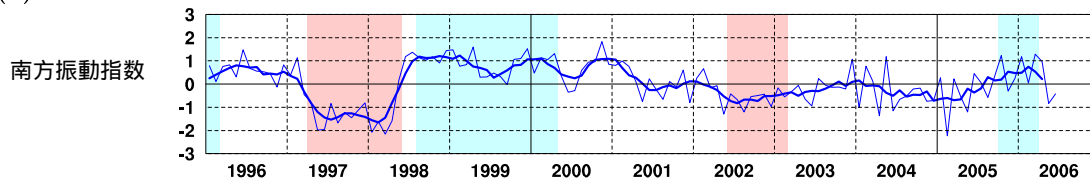
図1 エルニーニョ監視海域の海面水温の基準値との差( ^{\circ}\text{C} )(a)と南方振動指数(b)の推移(1996年1月~2006年6月)。折線は月平均値、滑らかな太線は5か月移動平均値を示す(海面水温の基準値はその年の前年までの30年間の各月の平均値、南方振動指数の年平均値は1971~2000年の30年平均値)。赤色の陰影はエルニーニョ現象の発生期間を、青色の陰影はラニーニャ現象の発生期間を示している。
