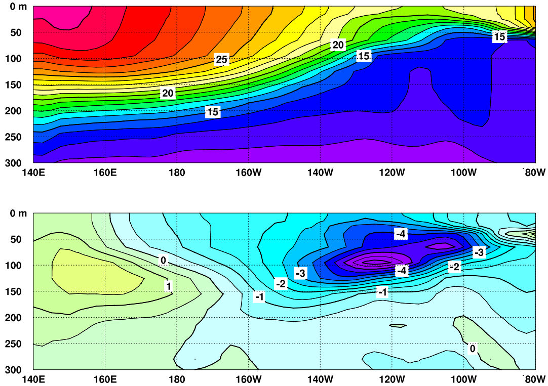
図3 2007年10月の太平洋の赤道に沿った水温(上)及び平年偏差(下)の断面図(海洋データ同化システムによる)。上図の等値線間隔は 1^{\circ}\text{C} 、下図の等値線間隔は 0.5^{\circ}\text{C} (平年値は1987~2006年の20年平均値)。
