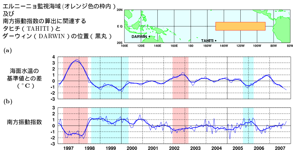
図1 エルニーニョ監視海域の海面水温の基準値との差( ^{\circ}\text{C} )(a)と南方振動指数(b)の推移(1997年1月~2007年10月)。折線は月平均値、滑らかな太線は5か月移動平均値を示す(海面水温の基準値はその年の前年までの30年間の各月の平均値、南方振動指数の平均値は1971~2000年の30年平均値)。赤色の陰影はエルニーニョ現象の発生期間を、青色の陰影はラニーニャ現象の発生期間を示している。
