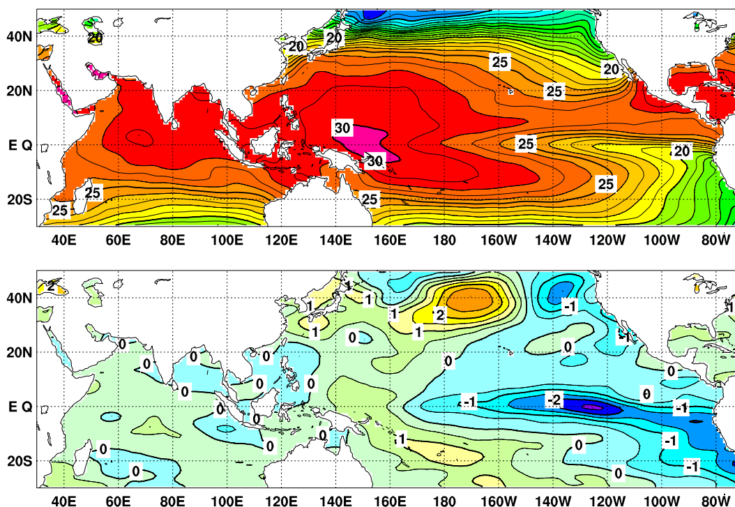
図 2 2007 年 10 月の海面水温図 ( 上 ) 及び平年偏差図 ( 下 )。海面水温図の太線は 5^{\circ}\text{C} 毎、細線は 1^{\circ}\text{C} 毎の、平年偏差図の太線は 1^{\circ}\text{C} 毎、細線は 0.5^{\circ}\text{C} 毎の等値線を示す ( 平年値は 1971 ~ 2000 年の 30 年平均値 )
