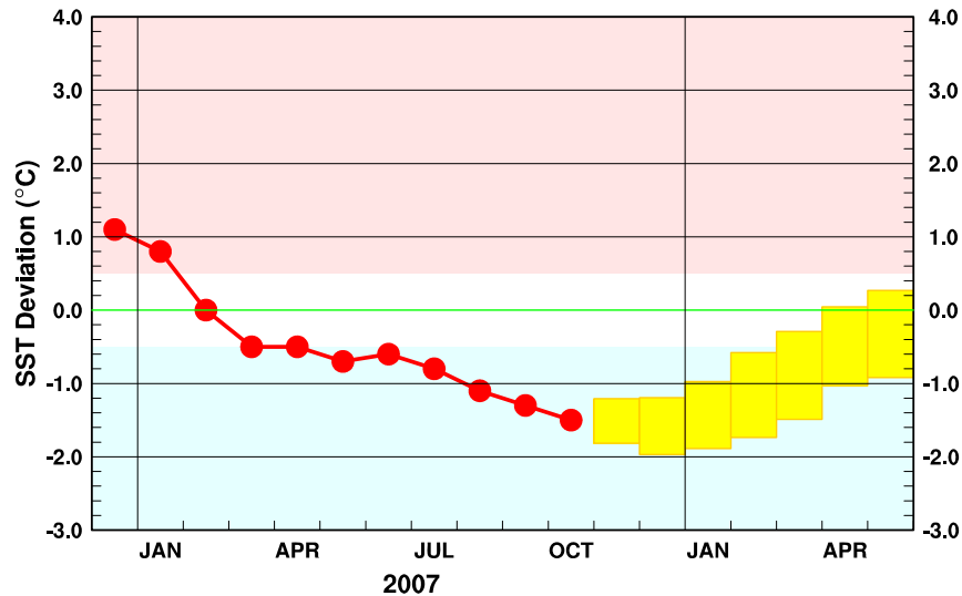
図9 エルニーニョ予測モデルによるエルニーニョ監視海域の海面水温予測。エルニーニョ監視海域の海面水温の基準値との差の先月までの推移(折れ線グラフ)と今後の予測(ボックス)を示す。各月のボックスは、海面水温の基準値との差が70%の確率で入る範囲を示す。(基準値はその年の前年までの30年間の各月の平均値)
