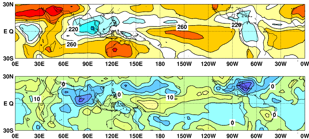
図 6 2007 年 10 月の外向き長波放射量 (OLR) ( 上 ) 及び平年偏差 ( 下 ) の分布図。OLR の値が小さいほど、対流活動が活発であることを示す。上図は 20\text{W}/\text{m}^2 毎、下図は 10\text{W}/\text{m}^2 毎に等値線を描いている ( 平年値は 1979 ~ 2004 年の 26 年平均値 )。OLR データは米国海洋大気庁 ( NOAA ) から提供されたものである。
