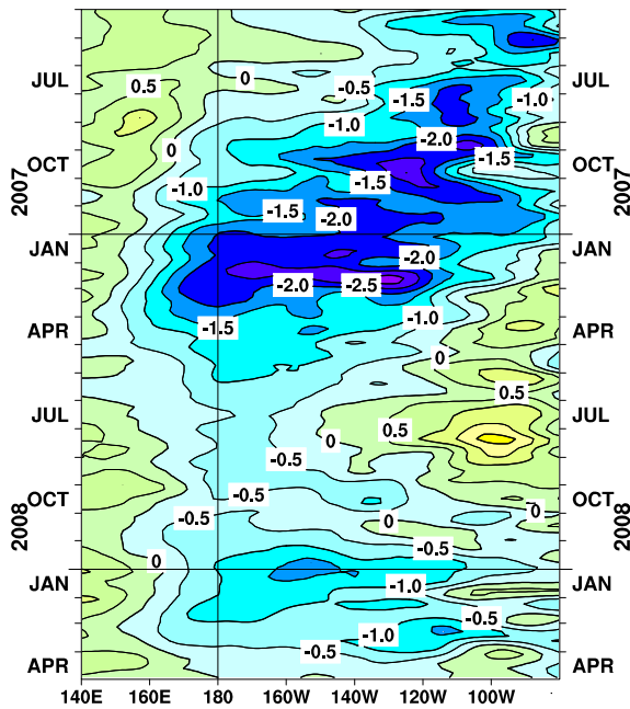
図4 太平洋の赤道に沿った海面水温年偏差の経度-時間断面図。等値線の間隔は 0.5^{\circ}\text{C} (年偏差は1971~2000年の30年平均値)。
