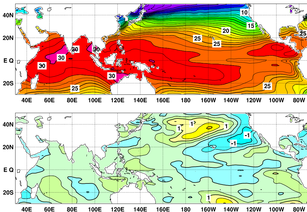
図 2 2009 年 4 月の海面水温図 ( 上 ) 及び平年偏差図 ( 下 )。海面水温図の太線は 5^{\circ}\text{C} 毎、細線は 1^{\circ}\text{C} 毎の、平年偏差図の太線は 1^{\circ}\text{C} 毎、細線は 0.5^{\circ}\text{C} 毎の等値線を示す ( 平年値は 1971 ~ 2000 年の 30 年平均値 )。
