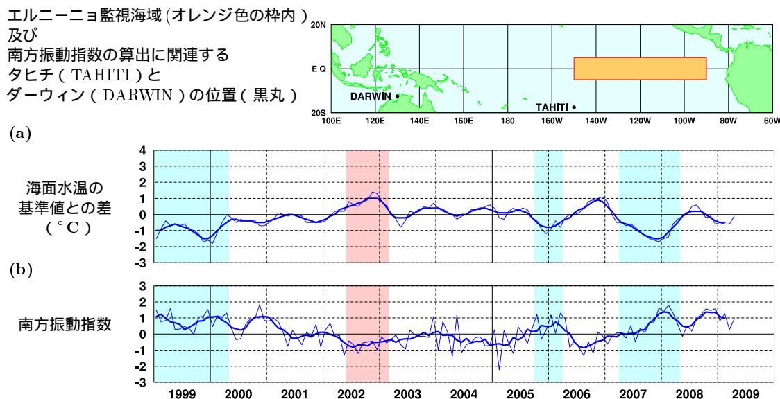
図1 エルニーニョ監視海域の海面水温の基準値との差( ^{\circ}\text{C} )(a)と南方振動指数(b)の推移(1999年1月~2009年4月)。折線は月平均値、滑らかな太線は5か月移動平均値を示す(海面水温の基準値はその年の前年までの30年間の各月の平均値、南方振動指数の年平均値は1971~2000年の30年平均値)。赤色の陰影はエルニーニョ現象の発生期間を、青色の陰影はラニーニャ現象の発生期間を示している。
