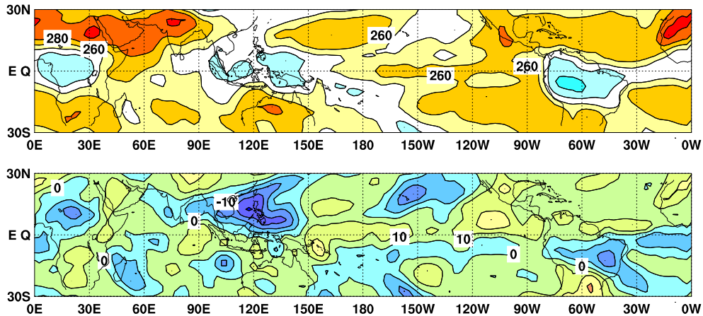
図 6 2009 年 4 月の外向き長波放射量 (OLR) ( 上 ) 及び年偏差 ( 下 ) の分布図。OLR の値が小さいほど、対流活動が活発であることを示す。上図は 20\text{W}/\text{m}^2 毎、下図は 10\text{W}/\text{m}^2 毎に等値線を描いている ( 平年値は 1979 ~ 2004 年の 26 年平均値 )。OLR データは米国海洋大気庁 ( NOAA ) から提供されたものである。
