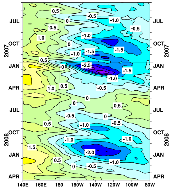
図5 太平洋の赤道に沿った海面から深度300mまでの平均水温年偏差の経度-時間断面図(海洋データ同化システムによる)。等値線の間隔は 0.5^{\circ}\text{C} (年偏差は1979~2004年の26年平均値)。
