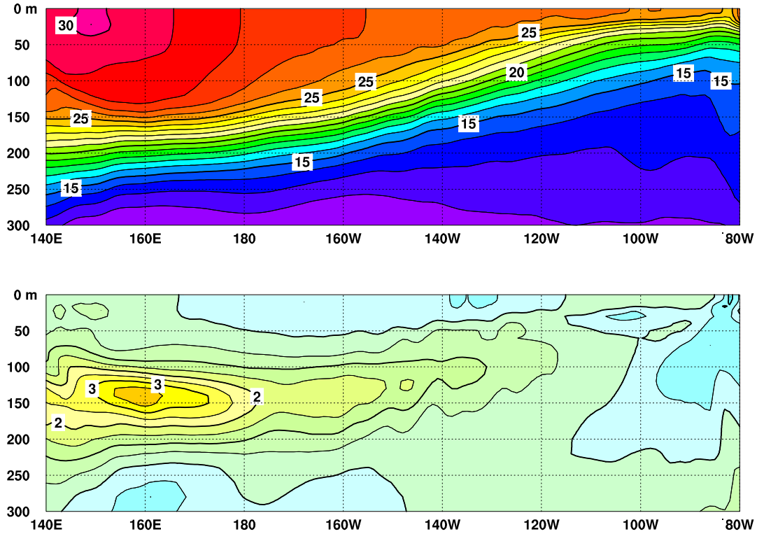
図3 2009年4月の太平洋の赤道に沿った水温(上)及び年偏差(下)の断面図(海洋データ同化システムによる)。上図の等値線間隔は 1^{\circ}\text{C} 、下図の等値線間隔は 0.5^{\circ}\text{C} (年偏差は1979~2004年の26年平均値)。
