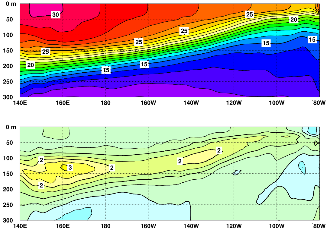
図3 2009年5月の太平洋の赤道に沿った水温(上)及び平年偏差(下)の断面図(海洋データ同化システムによる)。上図の等値線間隔は 1^{\circ}\text{C} 、下図の等値線間隔は 0.5^{\circ}\text{C} (平年値は1979~2004年の26年平均値)。
