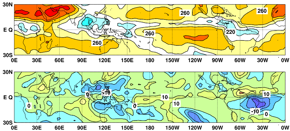
図 6 2009 年 5 月の外向き長波放射量 (OLR) ( 上 ) 及び平年偏差 ( 下 ) の分布図。OLR の値が小さいほど、対流活動が活発であることを示す。上図は 20\text{W}/\text{m}^2 毎、下図は 10\text{W}/\text{m}^2 毎に等値線を描いている ( 平年値は 1979 ~ 2004 年の 26 年平均値 )。OLR データは米国海洋大気庁 ( NOAA ) から提供されたものである。
