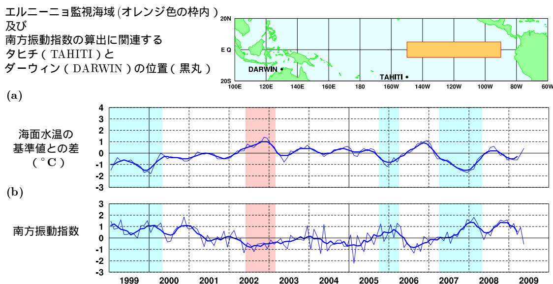
図1 エルニーニョ監視海域の海面水温の基準値との差( ^{\circ}\text{C} )(a)と南方振動指数(b)の推移(1999年1月~2009年5月)。折線は月平均値、滑らかな太線は5か月移動平均値を示す(海面水温の基準値はその年の前年までの30年間の各月の平均値、南方振動指数の年平均値は1971~2000年の30年平均値)。赤色の陰影はエルニーニョ現象の発生期間を、青色の陰影はラニーニャ現象の発生期間を示している。
