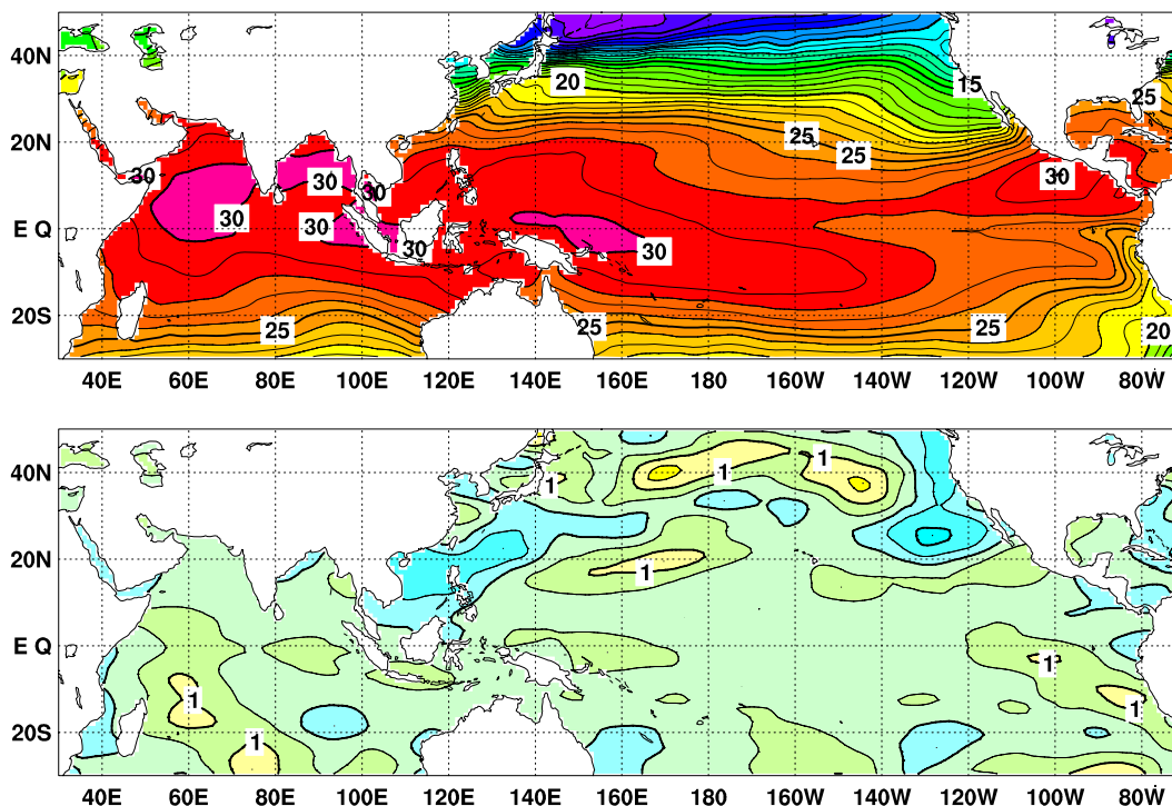
図 2 2009 年 5 月の海面水温図 ( 上 ) 及び平年偏差図 ( 下 )。海面水温図の太線は 5^{\circ}\text{C} 毎、細線は 1^{\circ}\text{C} 毎の、平年偏差図の太線は 1^{\circ}\text{C} 毎、細線は 0.5^{\circ}\text{C} 毎の等値線を示す ( 平年値は 1971 ~ 2000 年の 30 年平均値 )。
