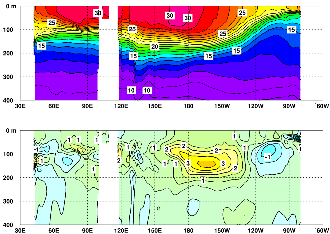
図 3 2009 年 10 月のインド洋から太平洋の赤道に沿った水温 ( 上 ) 及び 年 間 偏 差 ( 下 ) の 断 面 図
