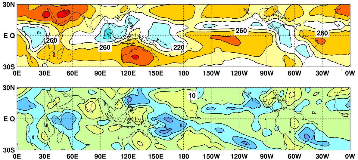
図6 外向き長波放射量 (OLR) (上) 及び年偏差 (下) の分布図 (2009 年 10 月)
