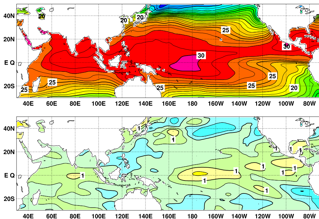
図 2 2009 年 10 月の海面水温図 ( 上 ) 及び 年 間 偏 差 図 ( 下 )
