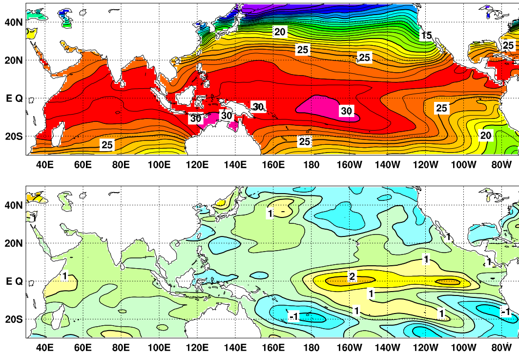
図 2 2009 年 12 月の海面水温図 ( 上 ) 及び 年 平 年 偏 差 図 ( 下 )
