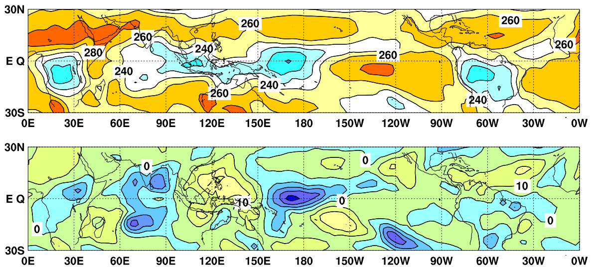
図6 外向き長波放射量 (OLR) (上) 及び年偏差 (下) の分布図 (2009 年 12 月)
