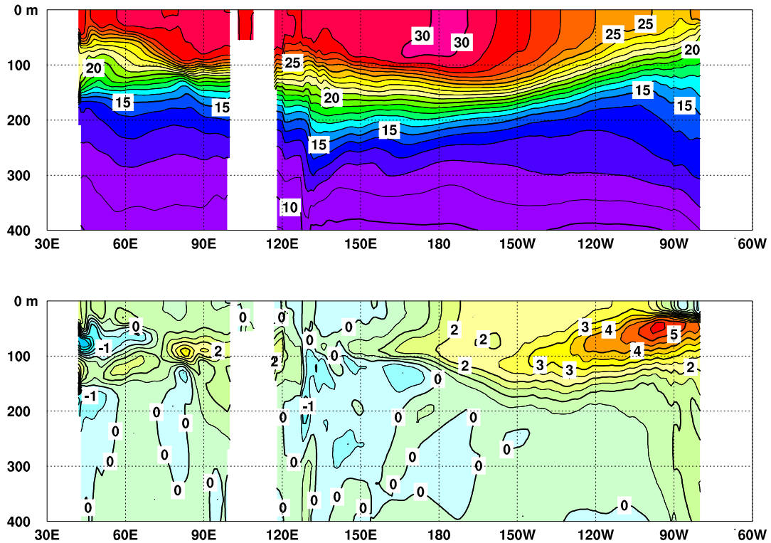
図 3 2009 年 12 月 の イ ン ド 洋 か ら 太 平 洋 の 赤 道 に 沿 っ た 水 温 ( 上 ) 及 び 年 平 年 偏 差 ( 下 ) の 断 面 図
