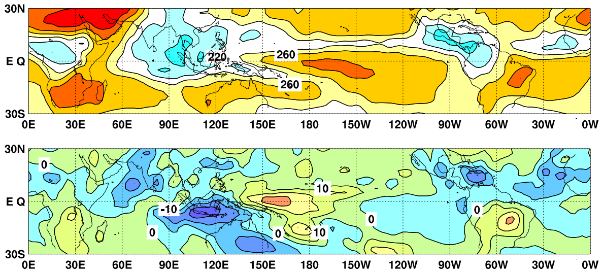
図6 外向き長波放射量 (OLR) (上) 及び年偏差 (下) の分布図 (2010 年 9 月)
