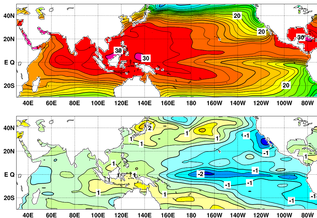
図 2 2010 年 9 月の海面水温図 ( 上 ) 及び 年 間 偏 差 図 ( 下 )
