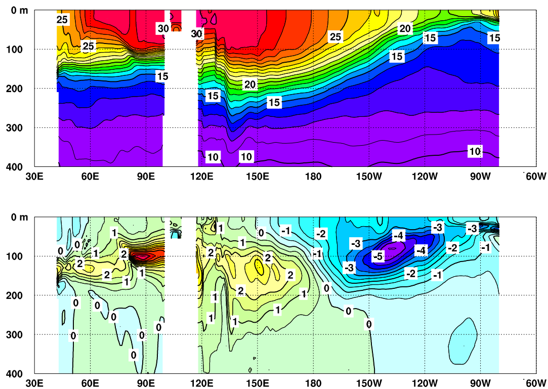
図 3 2010 年 9 月のインド 洋 から 太 平 洋 の 赤 道 に 沿 っ た 水 温 ( 上 ) 及 び 年 間 偏 差 ( 下 ) の 断 面 図
