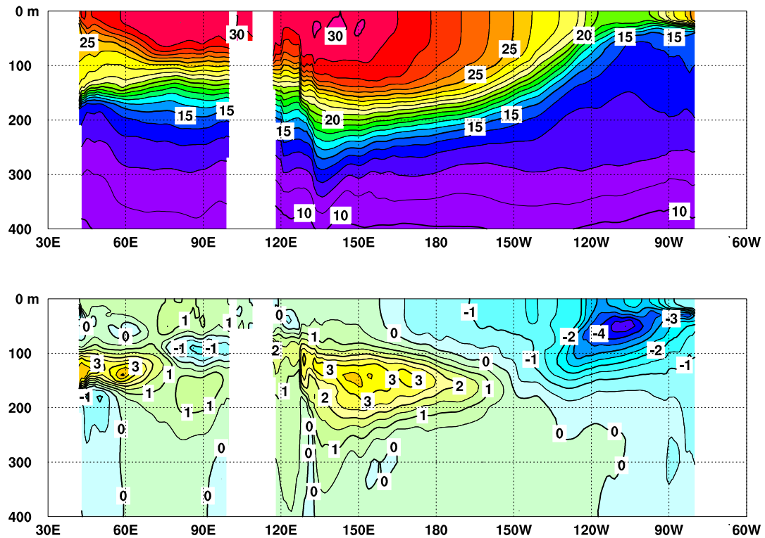
図 3 2011 年 11 月のインド洋から太平洋の赤道に沿った水温 ( 上 ) 及び平年偏差 ( 下 ) の断面図
