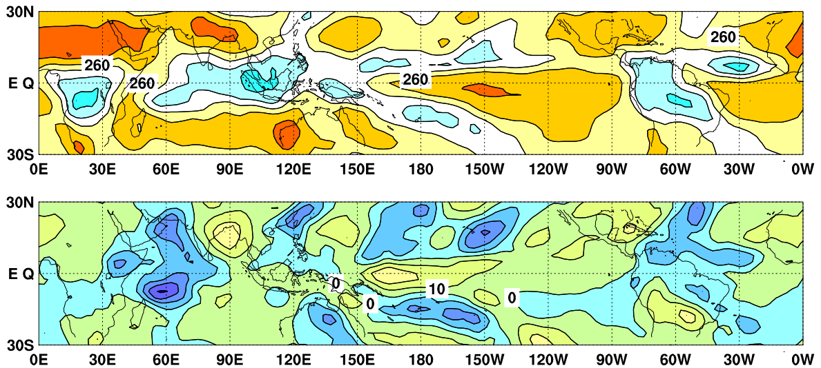
図6 外向き長波放射量 (OLR) (上) 及び年偏差 (下) の分布図 (2011 年 11 月)
