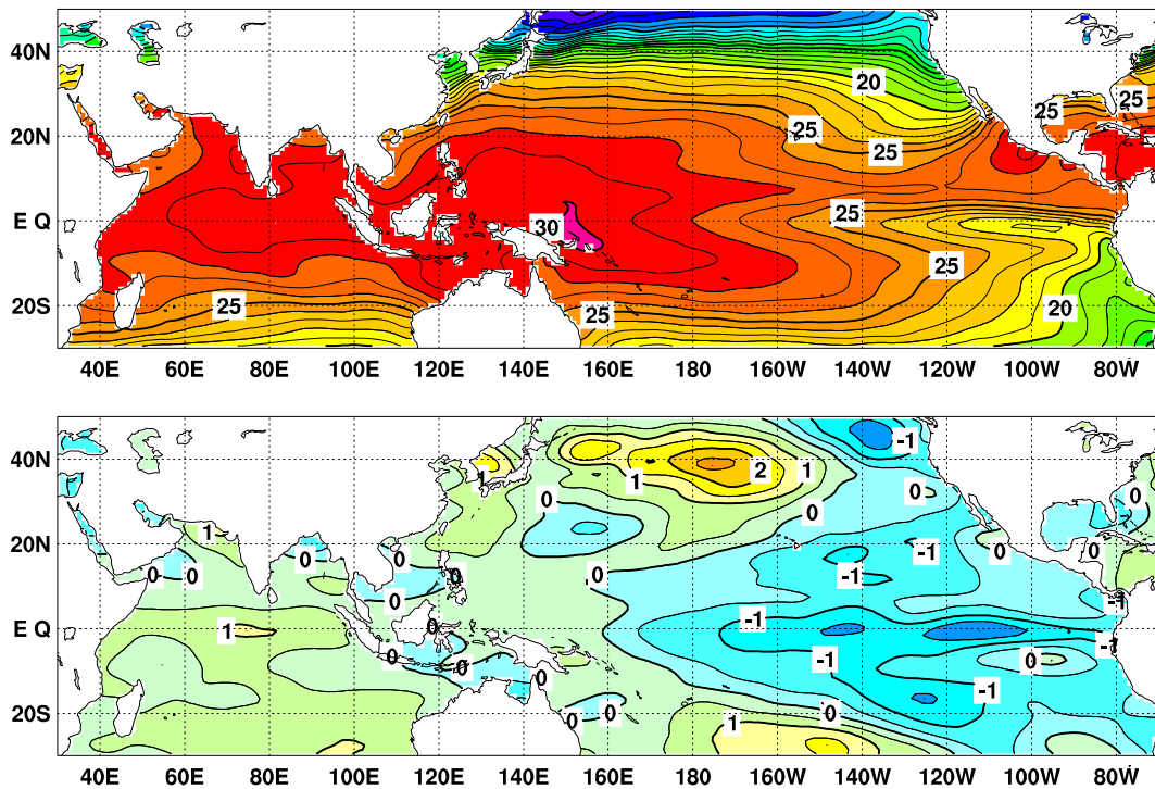
図 2 2011 年 11 月の海面水温図 ( 上 ) 及び平年偏差図 ( 下 )
