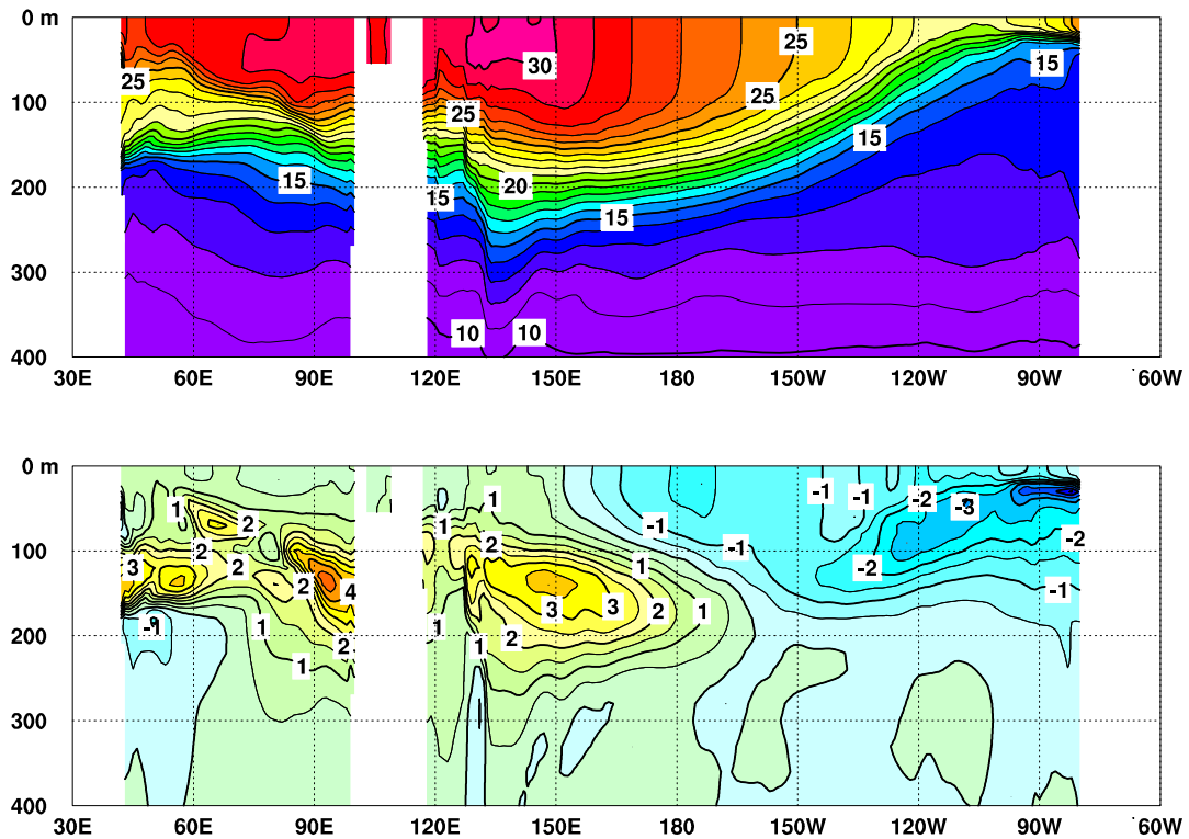
図 3 2011 年 12 月のインド洋から太平洋の赤道に沿った水温 ( 上 ) 及び平年偏差 ( 下 ) の断面図
