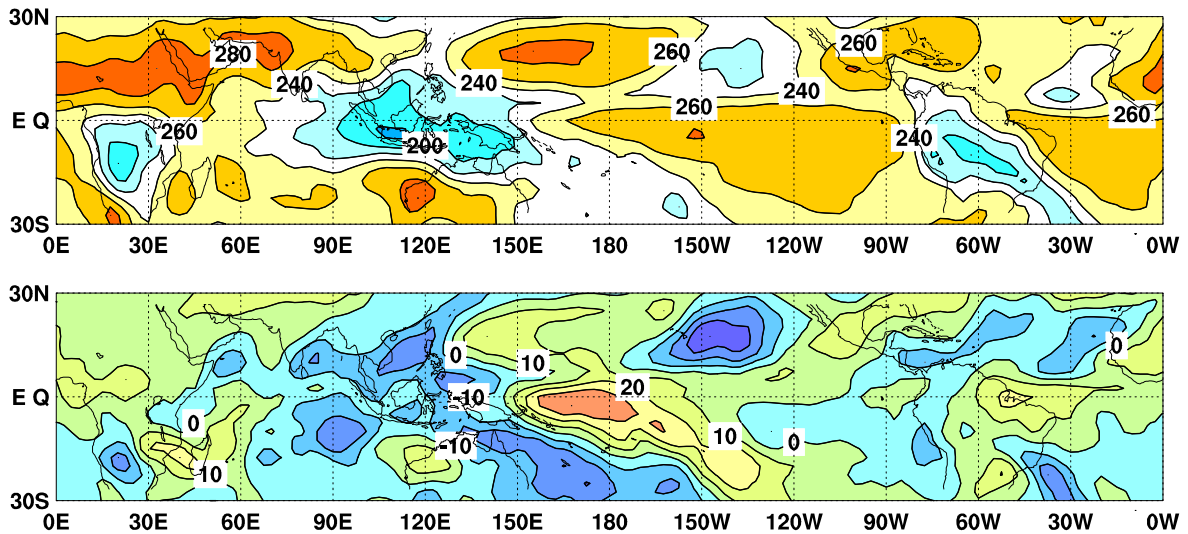
図6 外向き長波放射量 (OLR) (上) 及び年偏差 (下) の分布図 (2011 年 12 月)
