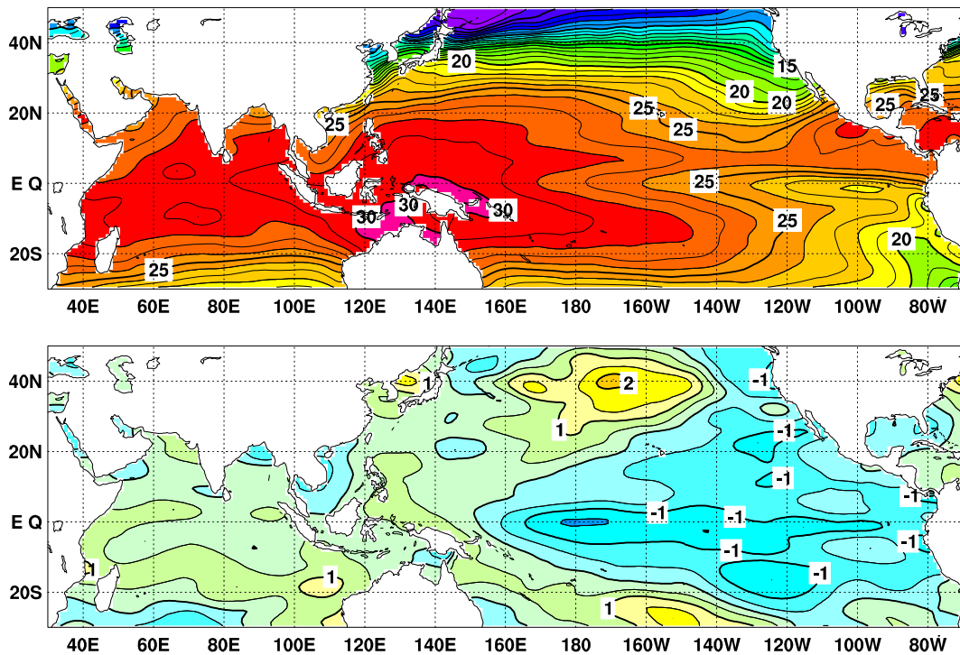
図 2 2011 年 12 月の海面水温図 ( 上 ) 及び平年偏差図 ( 下 )
