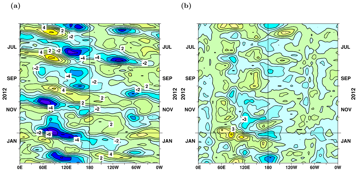
図8 赤道付近における対流圏上層 ( 200hPa ) の速度ポテンシャルの年偏差 ( a ) 及び対流圏下層 ( 850hPa ) の東西風速の年偏差 ( b ) の経度-時間断面図 ( a ) 等値線の間隔は 2 \times 10^6 \text{ m}^2/\text{s} で、平年よりも発散が強く、対流活動が活発な領域に青の陰影を、平年よりも発散が弱く、対流活動が不活発な領域に緑 ~ 黄 ~ 赤の陰影を施している。( b ) 等値線の間隔は 1.5 \text{ m/s} で、西風偏差の領域には緑 ~ 黄 ~ 赤の陰影を、東風偏差の領域には青の陰影を施している ( 両者の平年値は 1981 ~ 2010 年の 30 年平均値 )。
