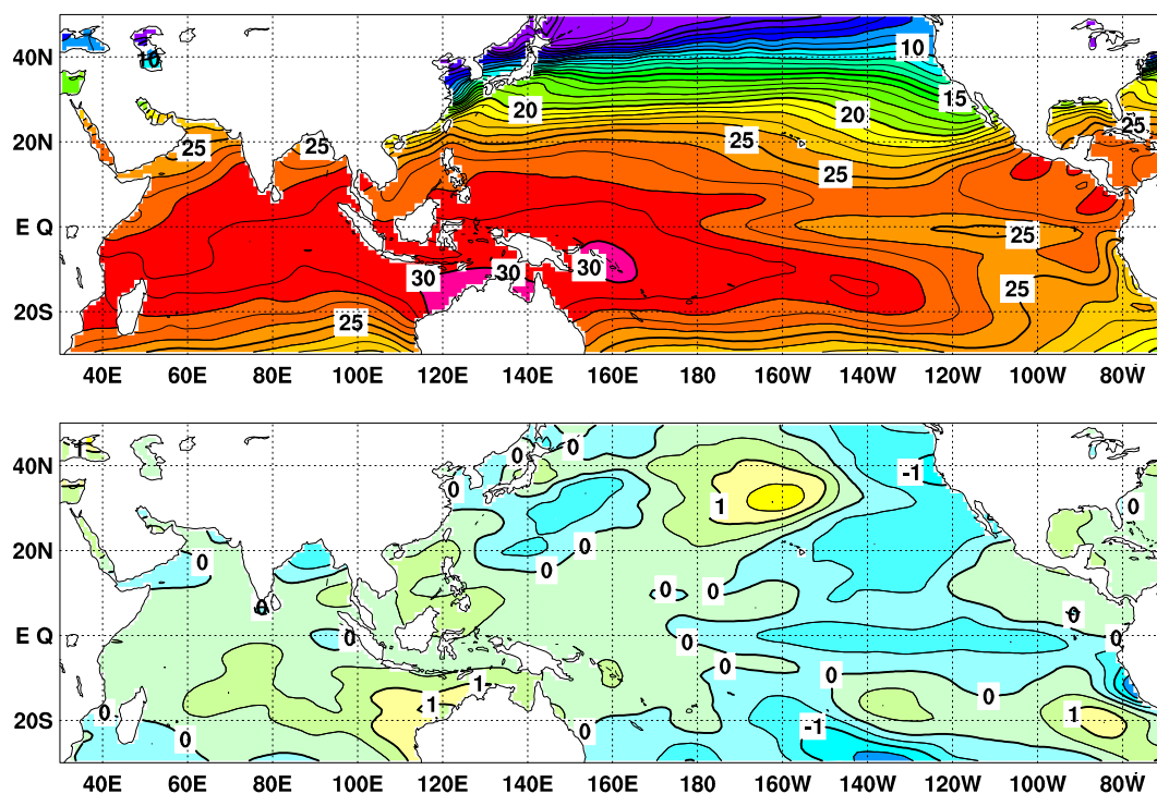
図 2 2013 年 2 月の海面水温図 ( 上 ) 及び平年偏差図 ( 下 )
