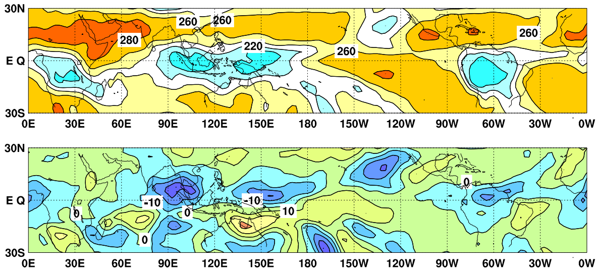
図6 外向き長波放射量 (OLR) (上) 及び年偏差 (下) の分布図 (2013 年 2 月)
