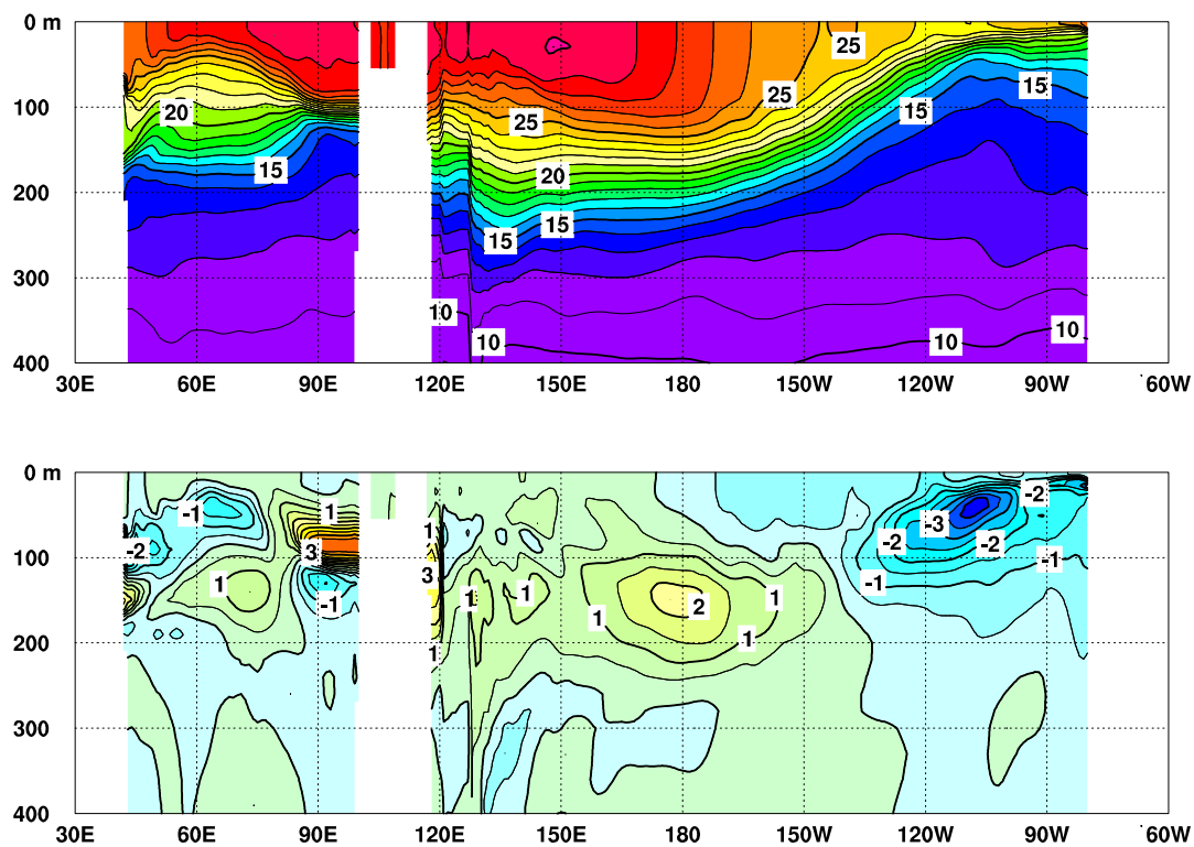
図 3 2013 年 2 月のインド洋から太平洋の赤道に沿った水温 ( 上 ) 及び平年偏差 ( 下 ) の断面図
