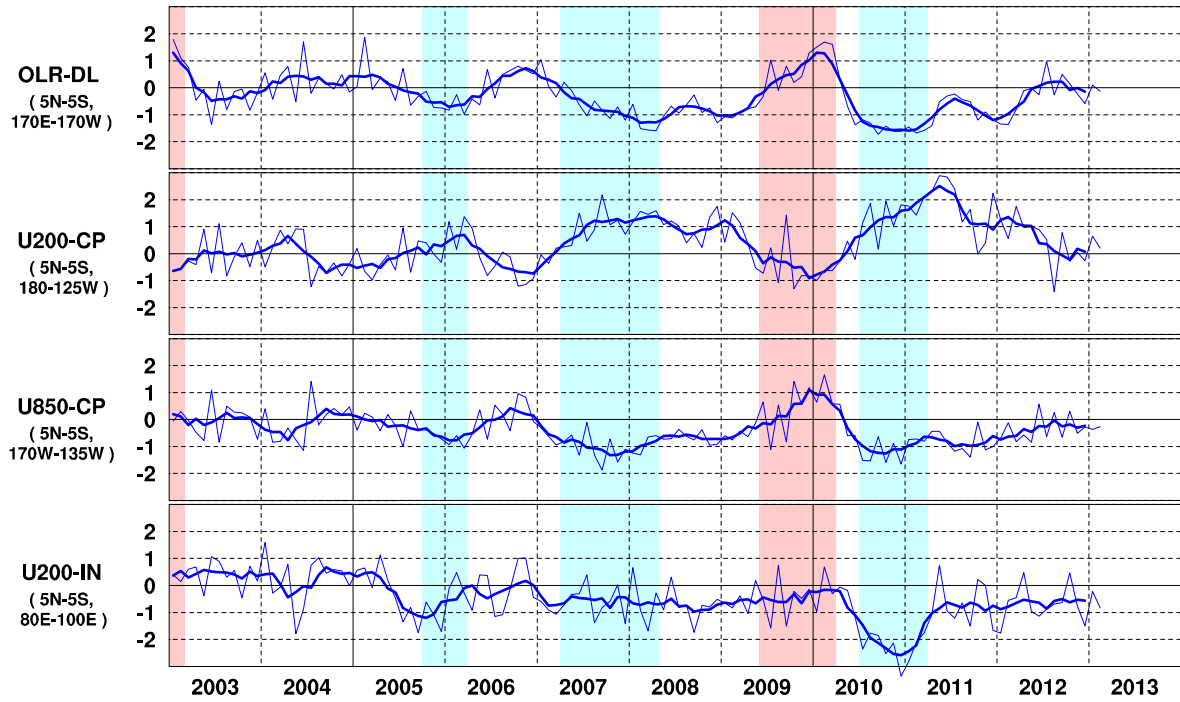
図7 日付変更線付近の OLR 指数 ( OLR-DL )、対流圏上層 ( 200hPa ) の赤道東西風指数 ( U200-CP )、対流圏下層 ( 850hPa ) の赤道東西風指数 ( U850-CP )、インド洋における対流圏上層 ( 200hPa ) の赤道東西風指数 ( U200-IN ) の時系列 ( 上から順に ) 折線は月平均値、滑らかな太線は 5 か月移動平均値を示す ( 平年値は 1981 ~ 2010 年の 30 年平均値 )。赤色の陰影はエルニーニョ現象の発生期間を、青色の陰影はラニーニャ現象の発生期間を示している。
