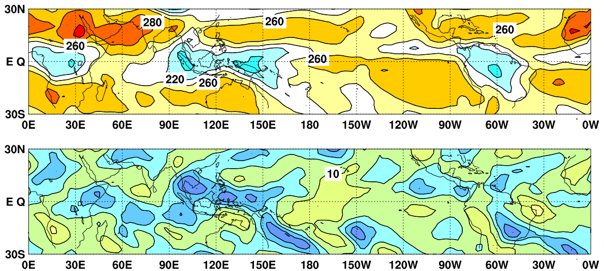
図 6 外向き長波放射量 ( OLR ) ( 上 ) 及び年偏差 ( 下 ) の分布図 ( 2013 年 4 月 )
