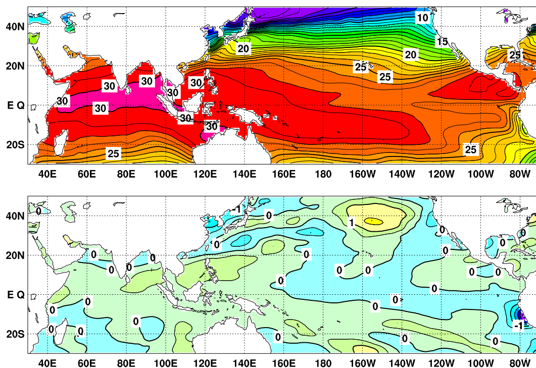
図 2 2013 年 4 月の海面水温図 ( 上 ) 及び平年偏差図 ( 下 )
