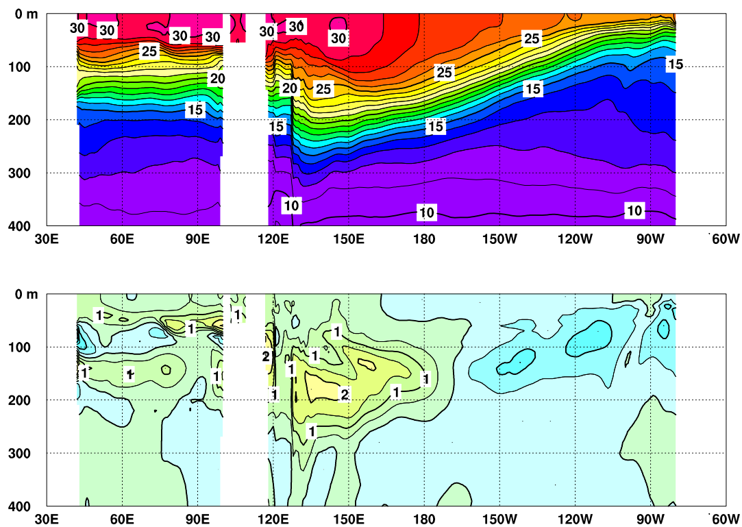
図 3 2013 年 4 月のインド洋から太平洋の赤道に沿った水温 ( 上 ) 及び平年偏差 ( 下 ) の断面図
