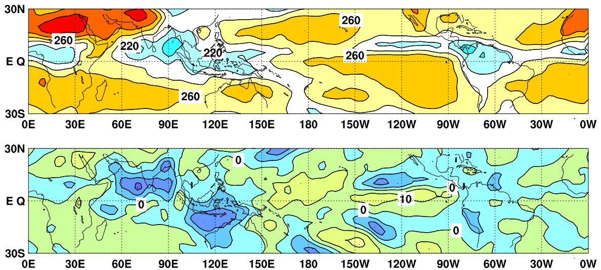
図 6 外向き長波放射量 ( OLR ) ( 上 ) 及び平年偏差 ( 下 ) の分布図 ( 2013 年 5 月 )
