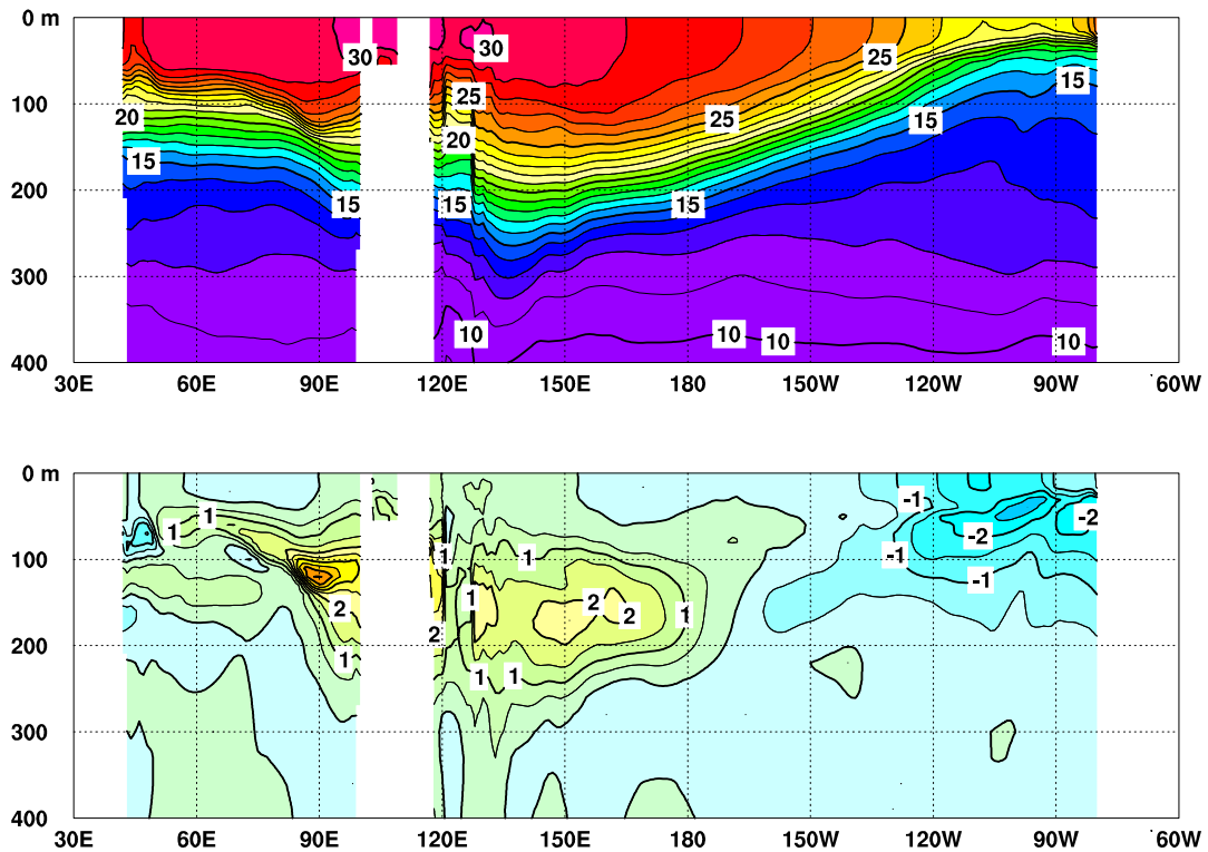
図 3 2013 年 5 月のインド洋から太平洋の赤道に沿った水温 ( 上 ) 及び平年偏差 ( 下 ) の断面図
