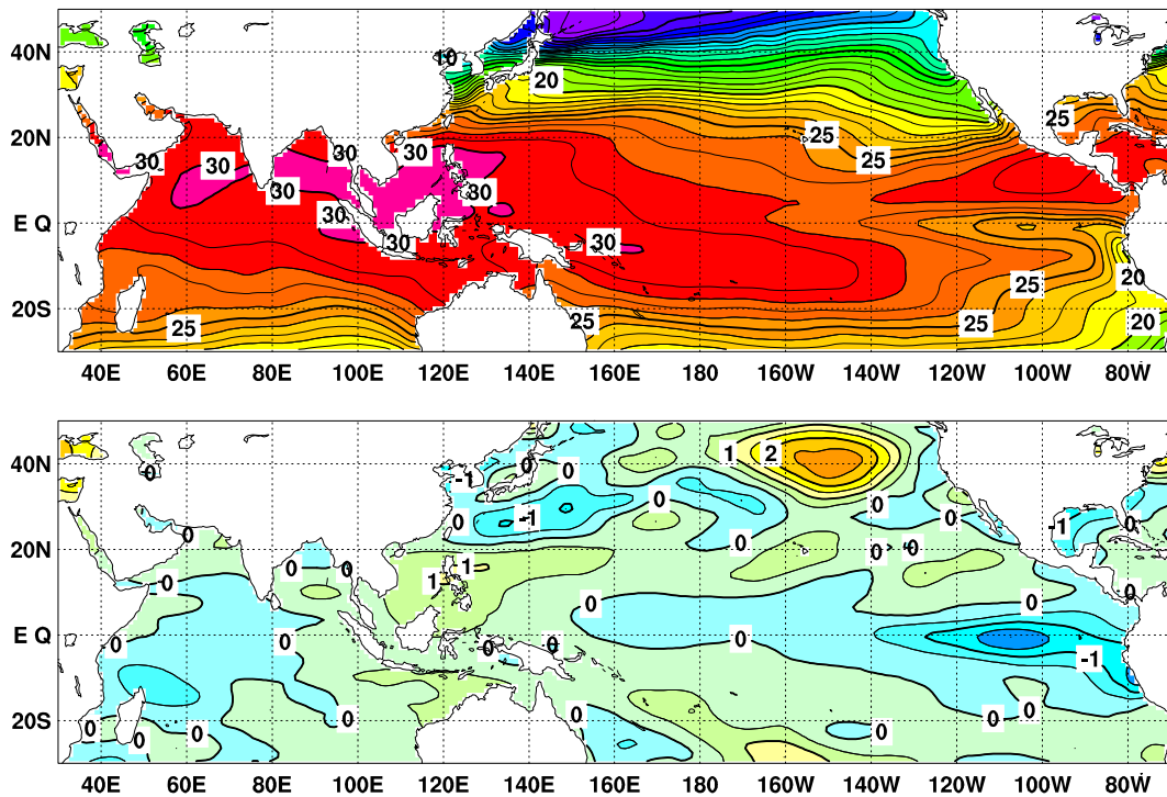
図 2 2013 年 5 月の海面水温図 ( 上 ) 及び平年偏差図 ( 下 )
