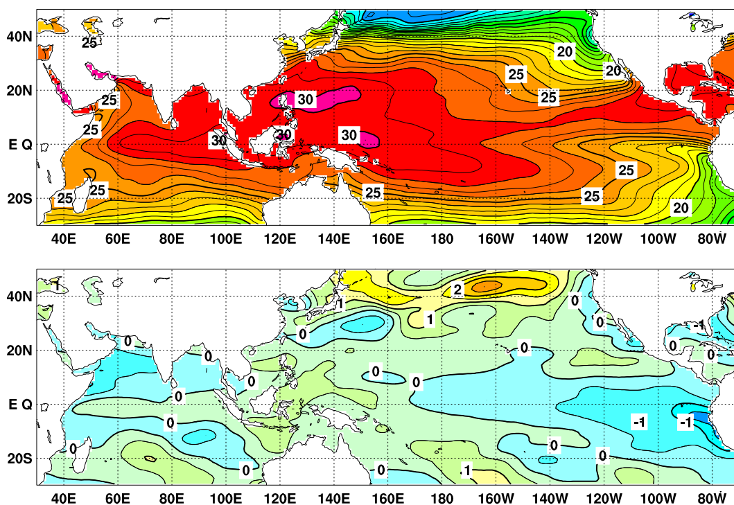
図 2 2013 年 7 月の海面水温図 ( 上 ) 及び平年偏差図 ( 下 )
