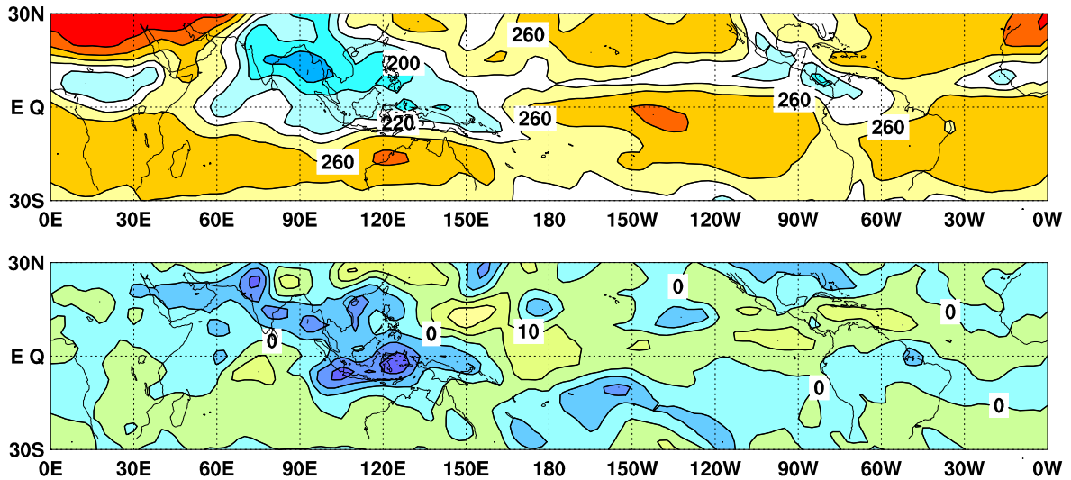
図6 外向き長波放射量(OLR)(上)及び年偏差(下)の分布図(2013年7月)
