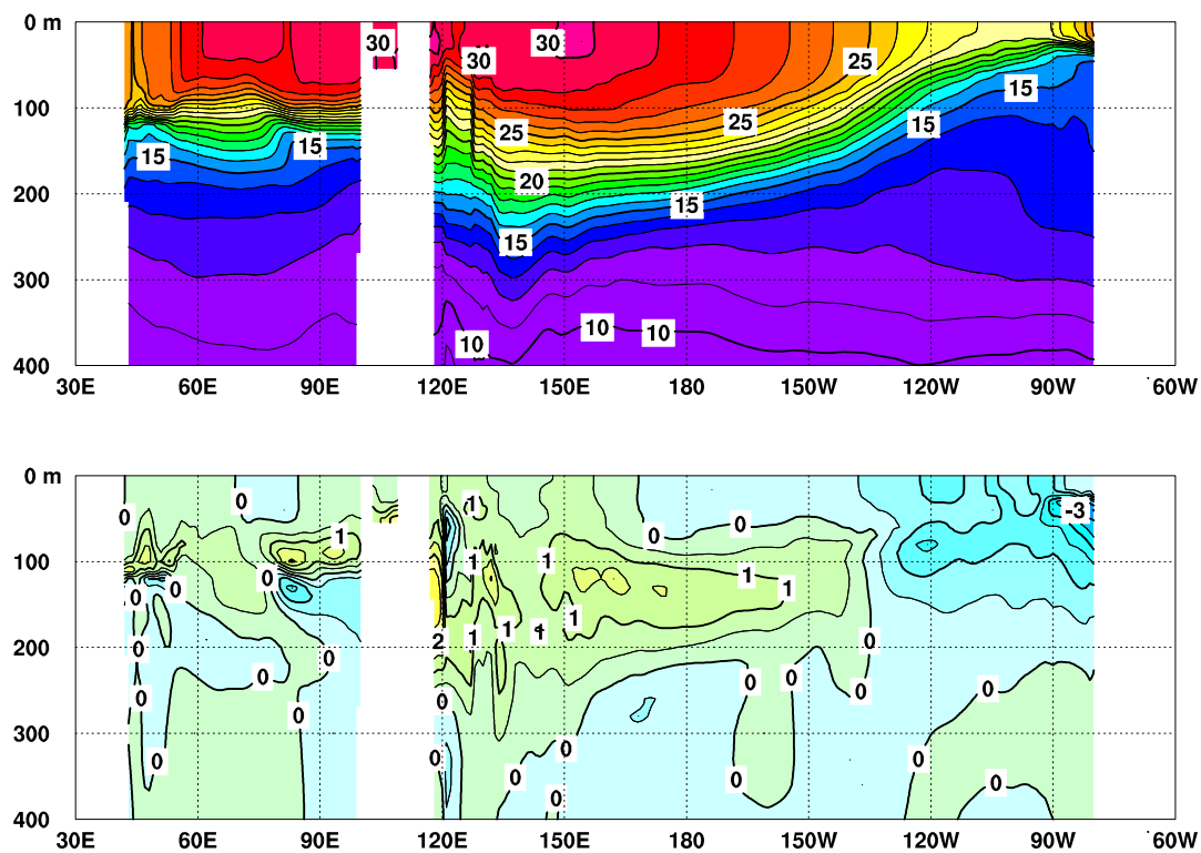
図 3 2013 年 7 月のインド洋から太平洋の赤道に沿った水温 ( 上 ) 及び平年偏差 ( 下 ) の断面図
