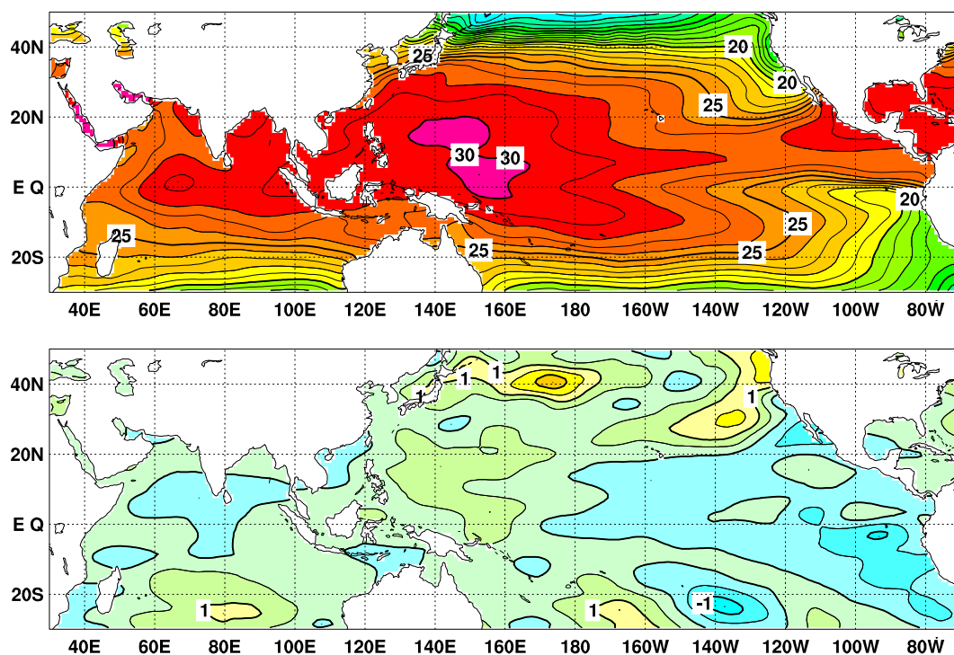
図 2 2013 年 9 月の海面水温図 ( 上 ) 及び平年偏差図 ( 下 )
