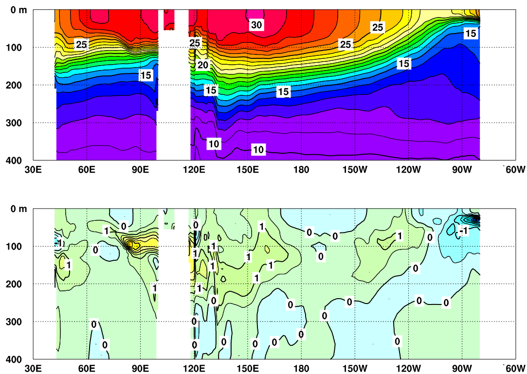
図 3 2013 年 9 月のインド洋から太平洋の赤道に沿った水温 ( 上 ) 及び平年偏差 ( 下 ) の断面図
