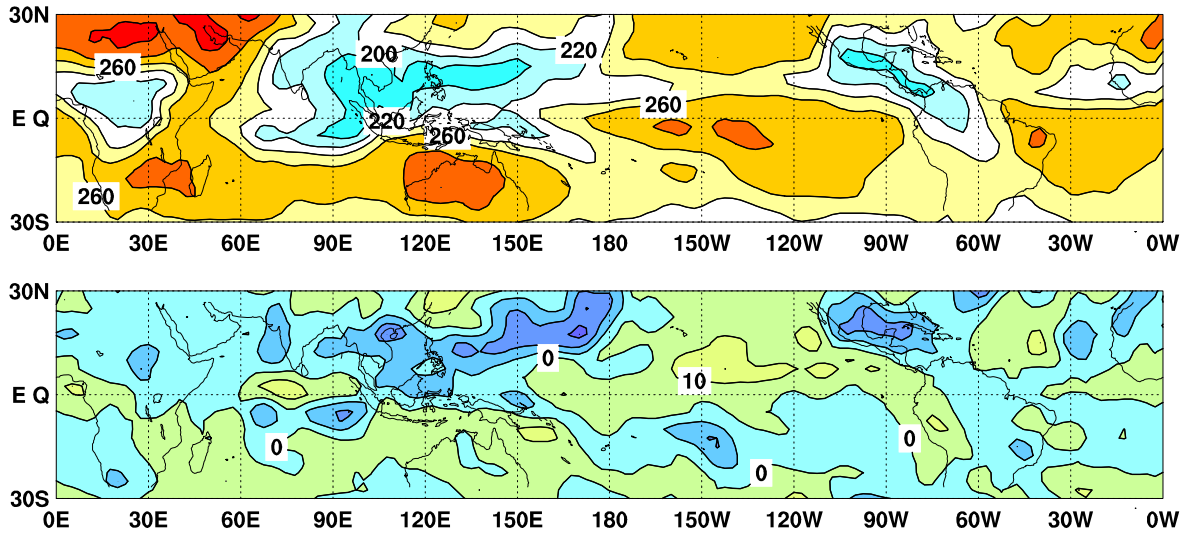
図6 外向き長波放射量 (OLR) (上) 及び年偏差 (下) の分布図 (2013 年 9 月)
