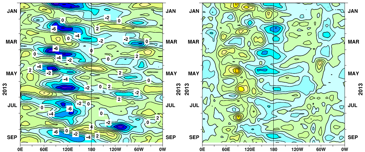
図8 赤道付近における対流圏上層 ( 200hPa ) の速度ポテンシャルの年平均偏差 ( a ) 及び対流圏下層 ( 850hPa ) の東西風速の年平均偏差 ( b ) の経度-時間断面図
