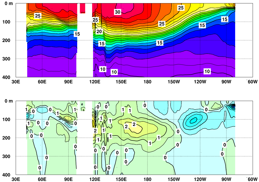
図 3 2013 年 10 月のインド洋から太平洋の赤道に沿った水温 ( 上 ) 及び平年偏差 ( 下 ) の断面図
