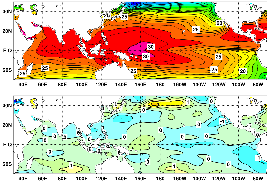
図 2 2013 年 10 月の海面水温図 ( 上 ) 及び平年偏差図 ( 下 )
