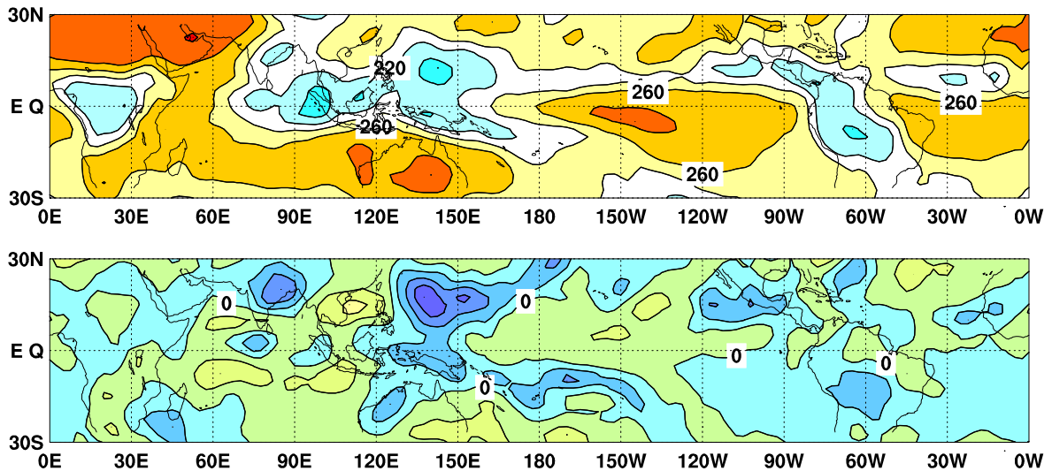
図6 外向き長波放射量 (OLR) (上) 及び年偏差 (下) の分布図 (2013 年 10 月)
