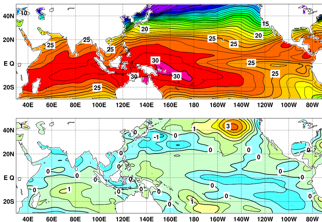
図 2 2014 年 1 月の海面水温図 ( 上 ) 及び平年偏差図 ( 下 )
