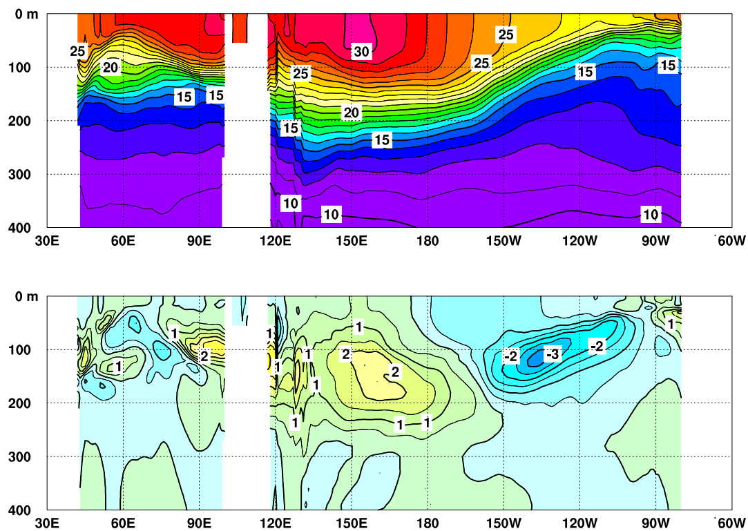
図 3 2014 年 1 月のインド洋から太平洋の赤道に沿った水温 ( 上 ) 及び平年偏差 ( 下 ) の断面図
