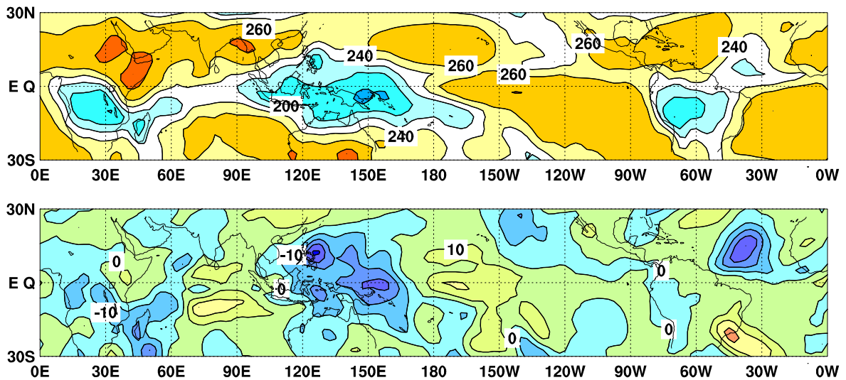
図6 外向き長波放射量 ( OLR ) ( 上 ) 及び平年偏差 ( 下 ) の分布図 ( 2014 年 1 月 )
