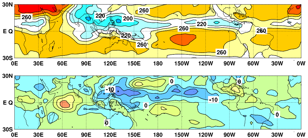
図6 外向き長波放射量(OLR)(上)及び年偏差(下)の分布図(2014年7月)
