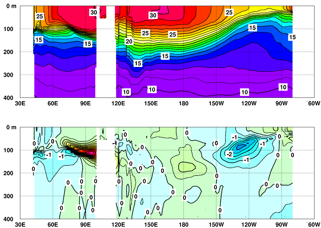
図 3 2014 年 7 月のインド洋から太平洋の赤道に沿った水温 ( 上 ) 及び平年偏差 ( 下 ) の断面図
