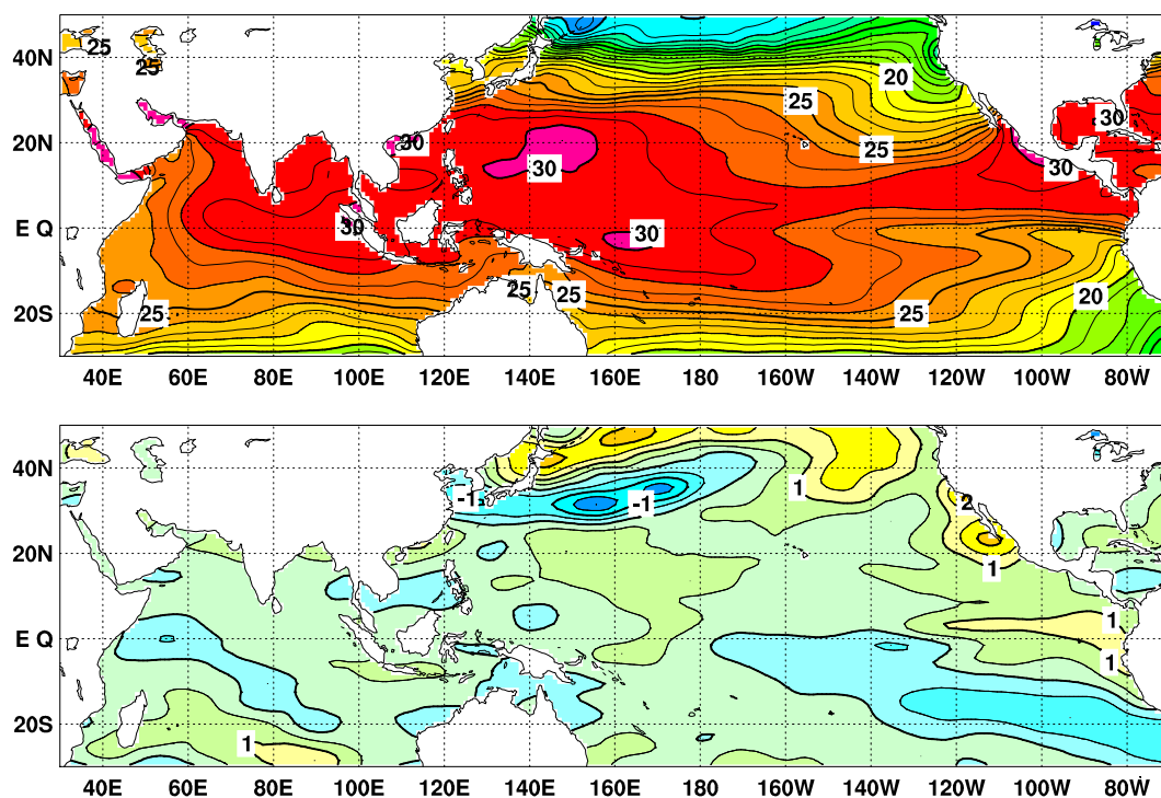
図 2 2014 年 7 月の海面水温図 ( 上 ) 及び平年偏差図 ( 下 )
