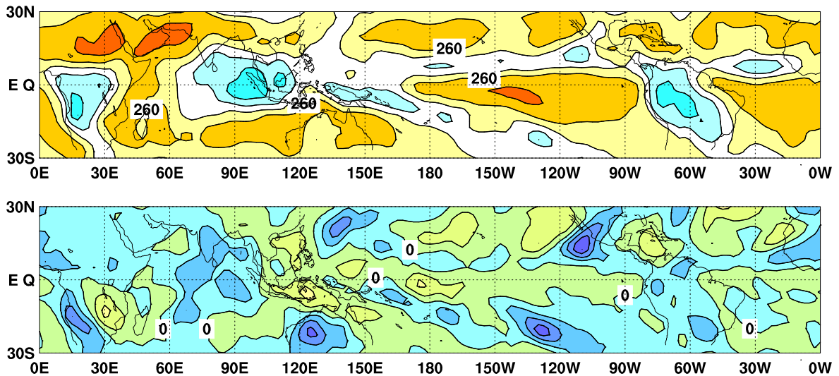
図6 外向き長波放射量 ( OLR ) ( 上 ) 及び年偏差 ( 下 ) の分布図 ( 2014 年 11 月 )
