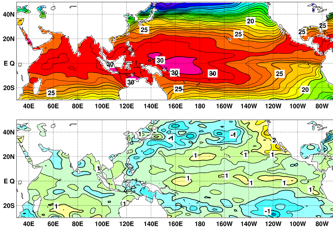
図 2 2014 年 11 月の海面水温図 ( 上 ) 及び平年偏差図 ( 下 )
