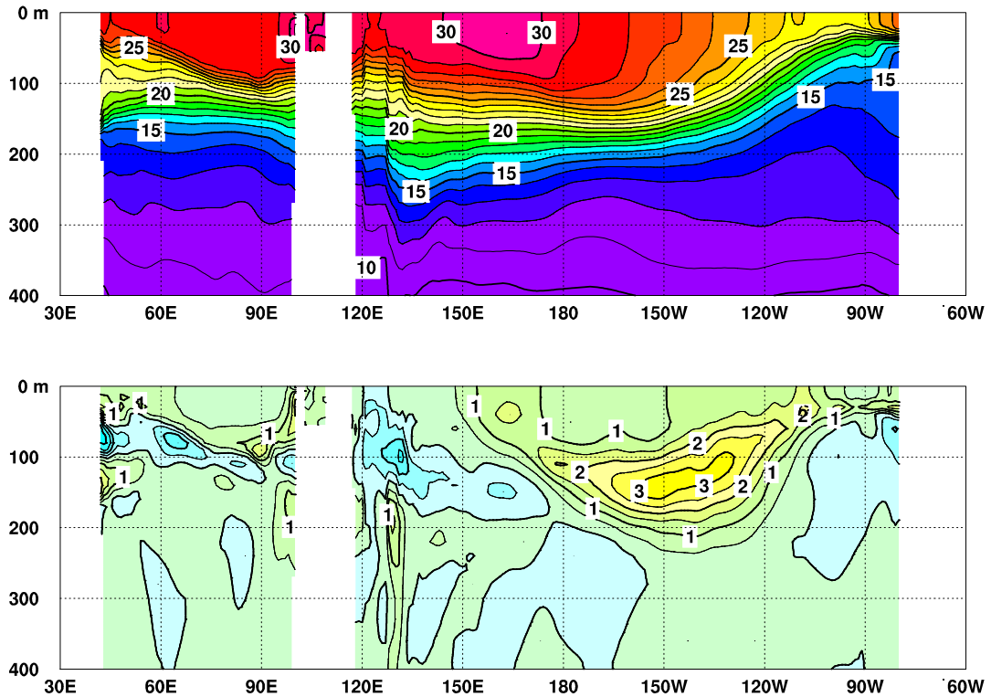
図 3 2014 年 11 月のインド洋から太平洋の赤道に沿った水温 ( 上 ) 及び平年偏差 ( 下 ) の断面図
