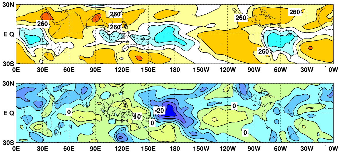
図6 外向き長波放射量 (OLR) (上) 及び年偏差 (下) の分布図 (2015 年 3 月)
