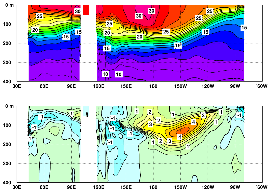
図 3 2015 年 3 月のインド洋から太平洋の赤道に沿った水温 (上) 及び平年偏差 (下) の断面図
