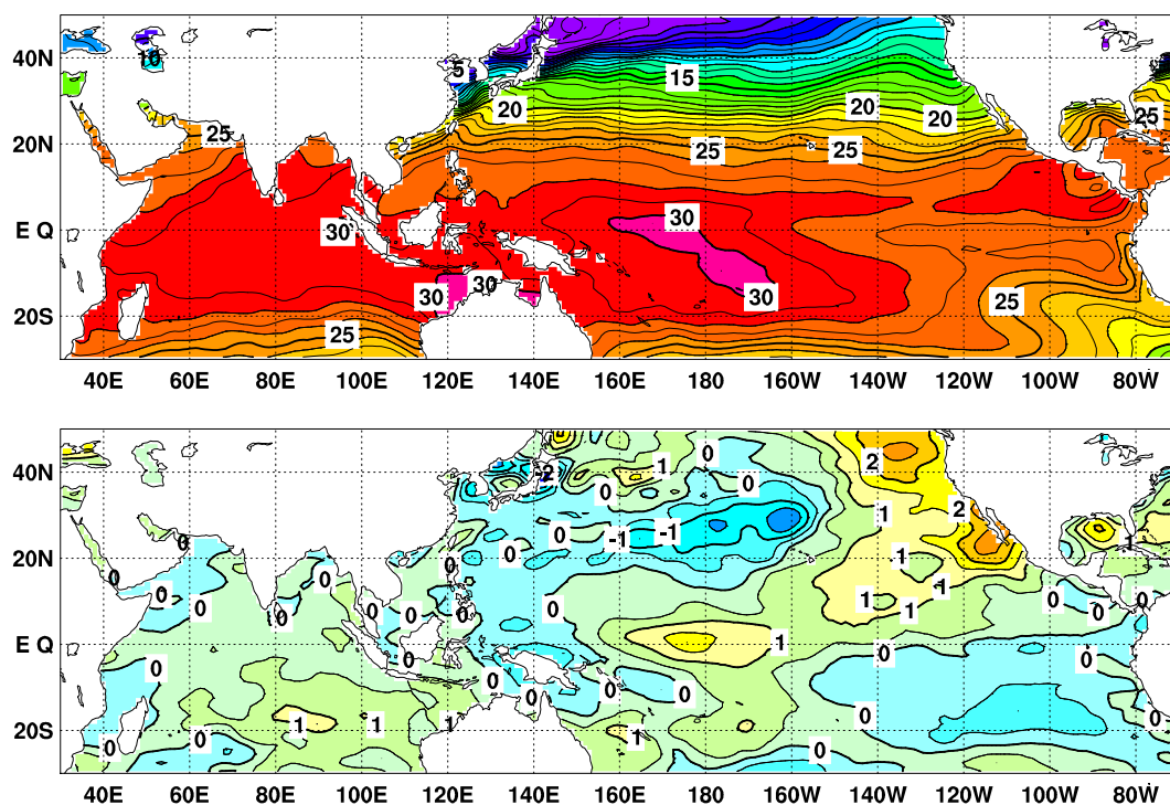
図 2 2015 年 3 月の海面水温図 (上) 及び平年偏差図 (下)
