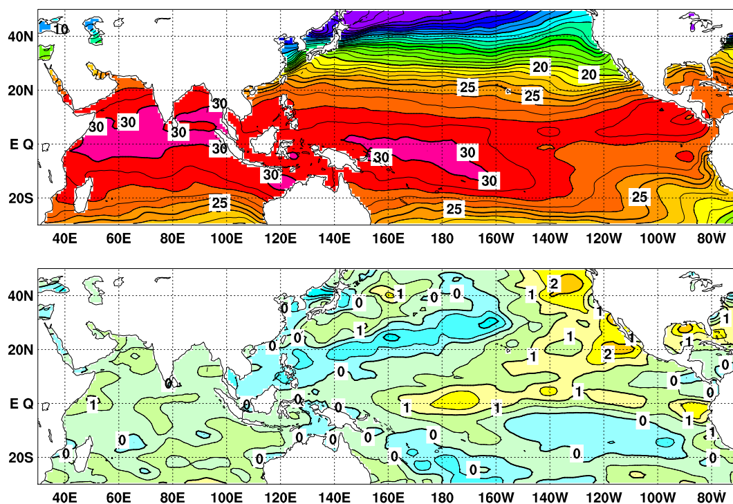
図 2 2015 年 4 月の海面水温図 ( 上 ) 及び平年偏差図 ( 下 )
