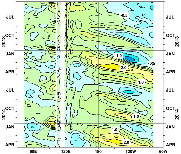
図5 インド洋から太平洋の赤道に沿った海面から深 度 300m までの平均水温年偏差の経度-時間断面図 太線は 1^{\circ}\text{C} 毎、細線は 0.5^{\circ}\text{C} 毎の等値線を示す（平 年値は 1981- 2010 年の 30 年平均値）。図中白く抜け ている部分は陸地である。
