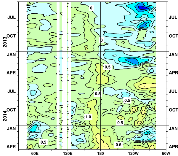
図4 インド洋から太平洋の赤道に沿った海面水温 年偏差の経度-時間断面図 太線は 1^{\circ}\text{C} 毎、細線は 0.5^{\circ}\text{C} 毎の等値線を示す（平 年値は 1981- 2010 年の 30 年平均値）。図中白く抜け ている部分は陸地である。
