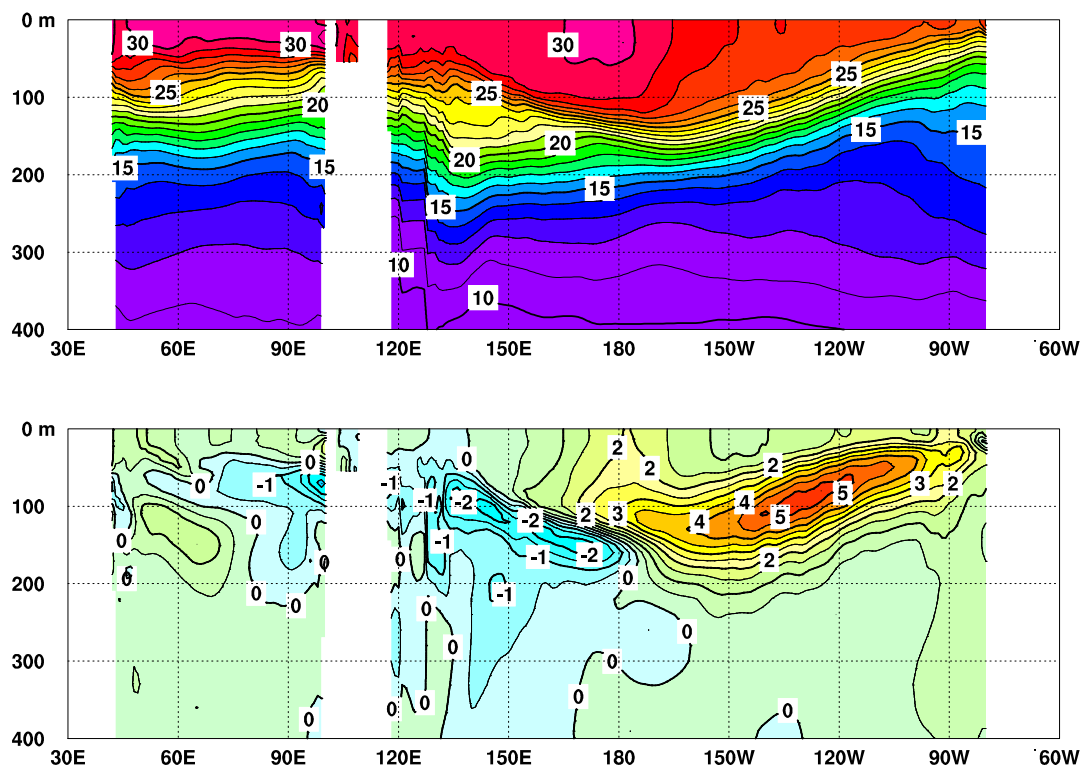
図 3 2015 年 4 月のインド洋から太平洋の赤道に沿った水温 ( 上 ) 及び平年偏差 ( 下 ) の断面図
