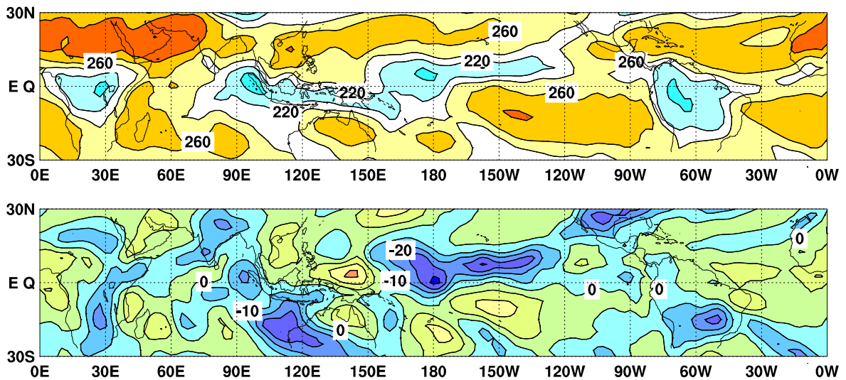
図6 外向き長波放射量 (OLR) (上) 及び平年偏差 (下) の分布図 (2015 年 4 月)
