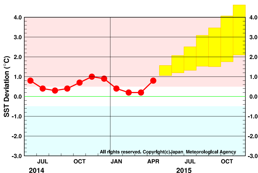
図 9 エルニーニョ監視海域の月平均海面水温の基準値との差の先月までの経過（折れ線グラフ）とエルニーニョ予測モデルから得られた今後の予測（ボックス）
