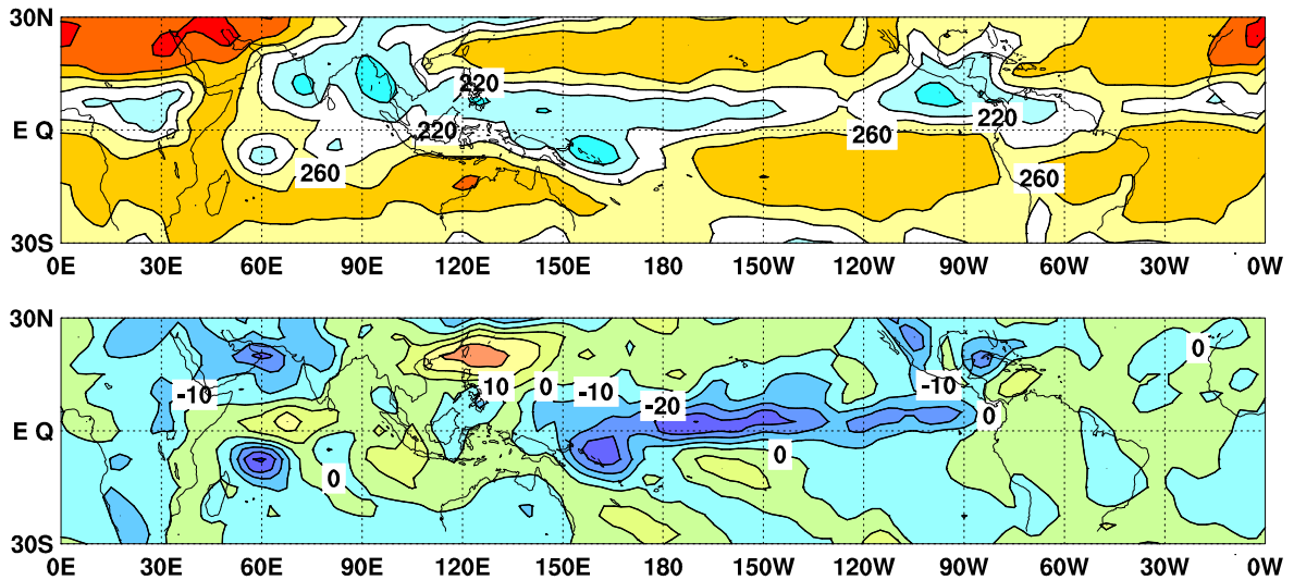
図6 外向き長波放射量 (OLR) (上) 及び年偏差 (下) の分布図 (2015 年 6 月)
