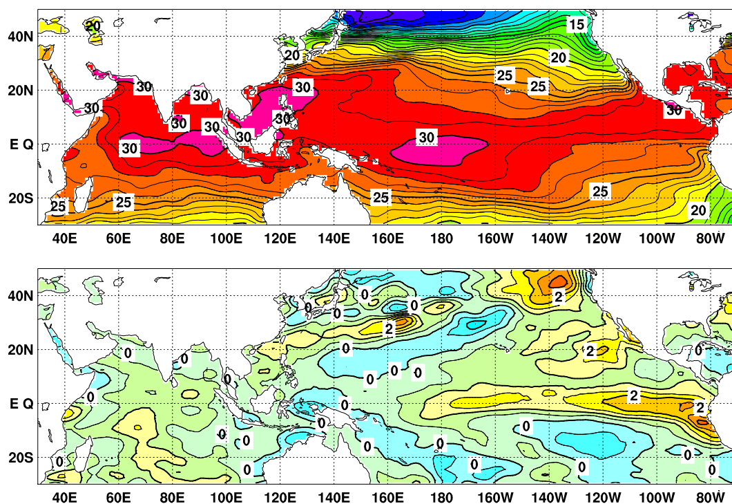
図 2 2015 年 6 月の海面水温図 ( 上 ) 及び平年偏差図 ( 下 )
