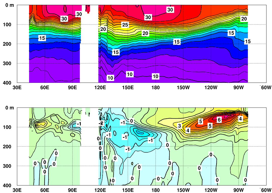
図 3 2015 年 6 月のインド洋から太平洋の赤道に沿った水温 ( 上 ) 及び平年偏差 ( 下 ) の断面図
