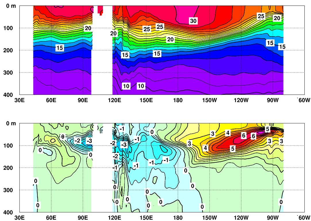
図 3 2015 年 10 月のインド洋から太平洋の赤道に沿った水温 ( 上 ) 及び平年偏差 ( 下 ) の断面図
