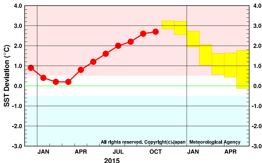
図 9 エルニーニョ監視海域の月平均海面水温の基準値との差の先月までの経過（折れ線グラフ）とエルニーニョ予測モデルから得られた今後の予測（ボックス） 各月のボックスは、海面水温の基準値との差が 70%の確率で入る範囲を示す。
