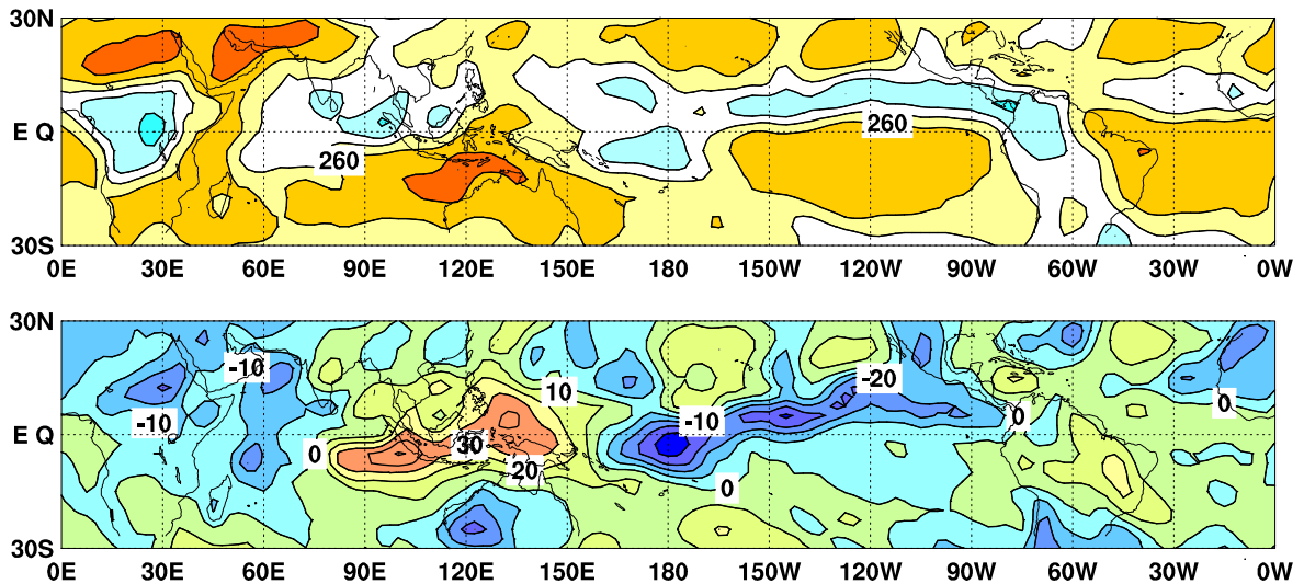
図6 外向き長波放射量 ( OLR ) ( 上 ) 及び年偏差 ( 下 ) の分布図 ( 2015 年 10 月 )
