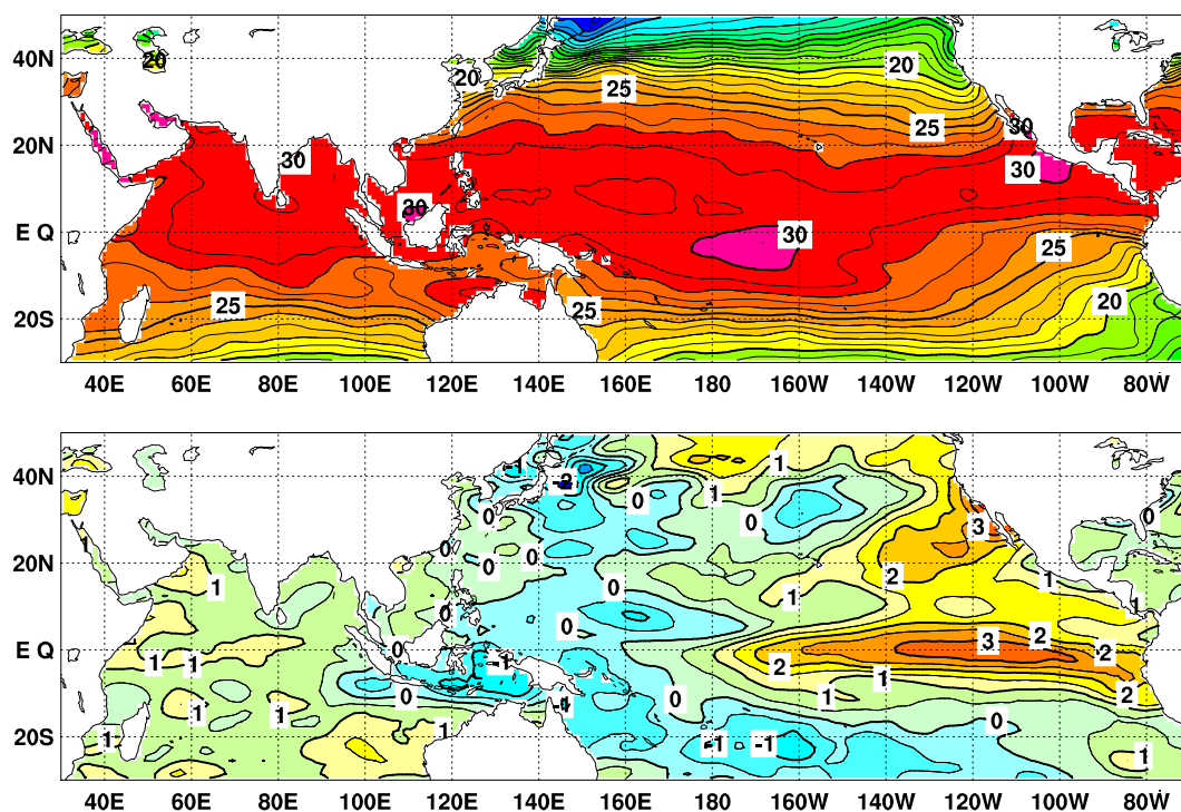
図 2 2015 年 10 月の海面水温図 ( 上 ) 及び平年偏差図 ( 下 )
