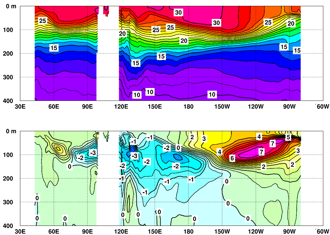
図3 2015年11月のインド洋から太平洋の赤道に沿った水温(上)及び年偏差(下)の断面図
