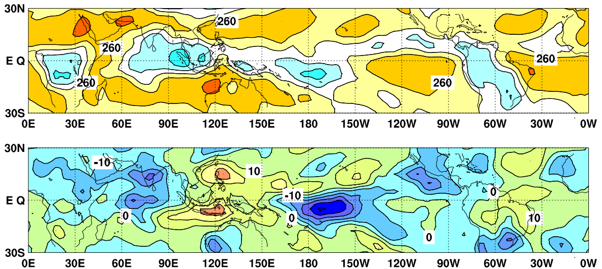
図6 外向き長波放射量 (OLR) (上) 及び年偏差 (下) の分布図 (2015年11月)
