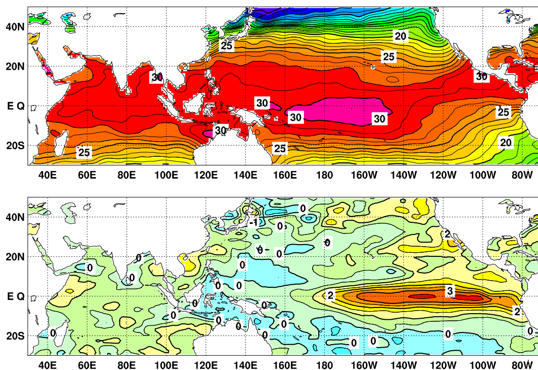
図2 2015年11月の海面水温図(上)及び年偏差図(下)
