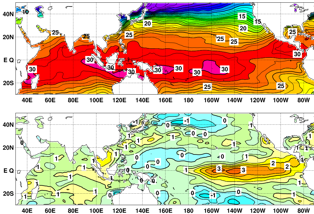
図2 2016年1月の海面水温図(上)及び平年偏差図(下)
