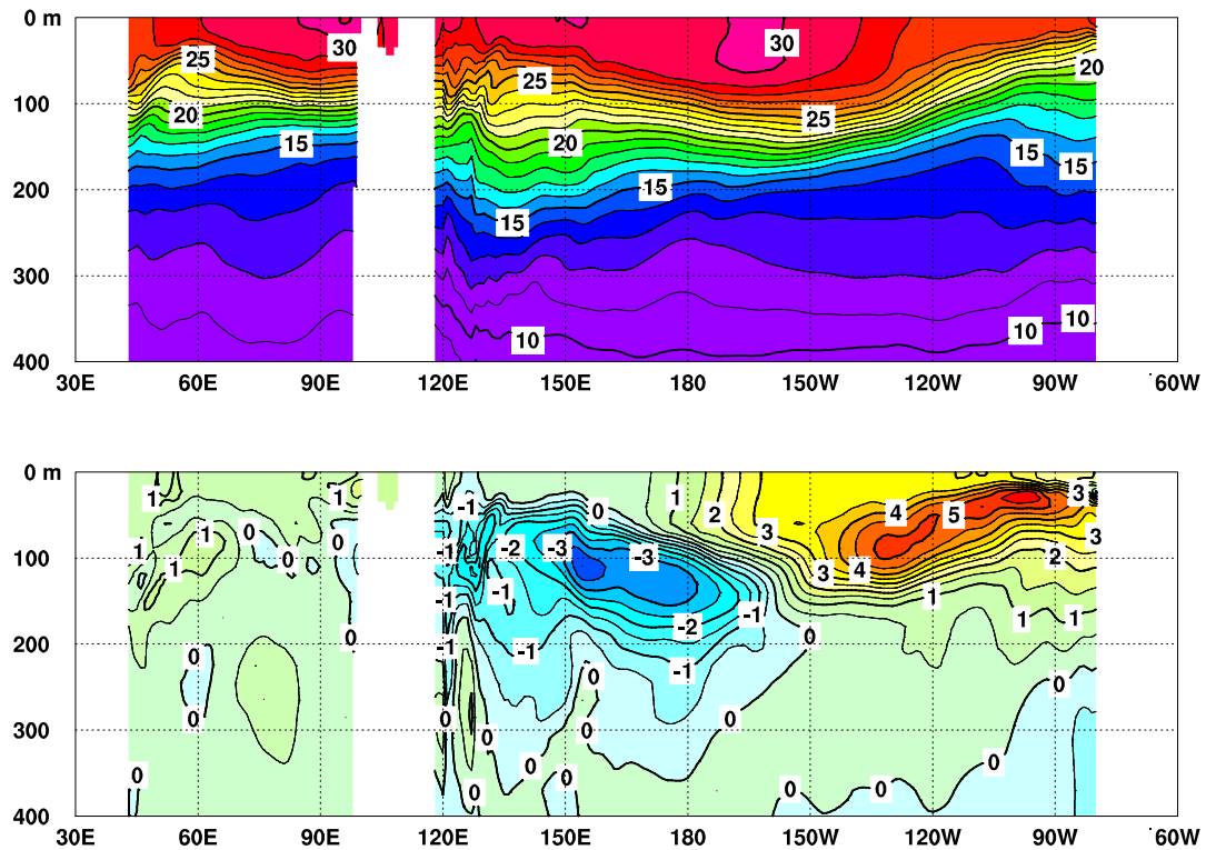
図3 2016年1月のインド洋から太平洋の赤道に沿った水温(上)及び平年偏差(下)の断面図
