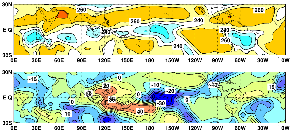
図6 外向き長波放射量 (OLR) (上) 及び年偏差 (下) の分布図 (2016年1月)
