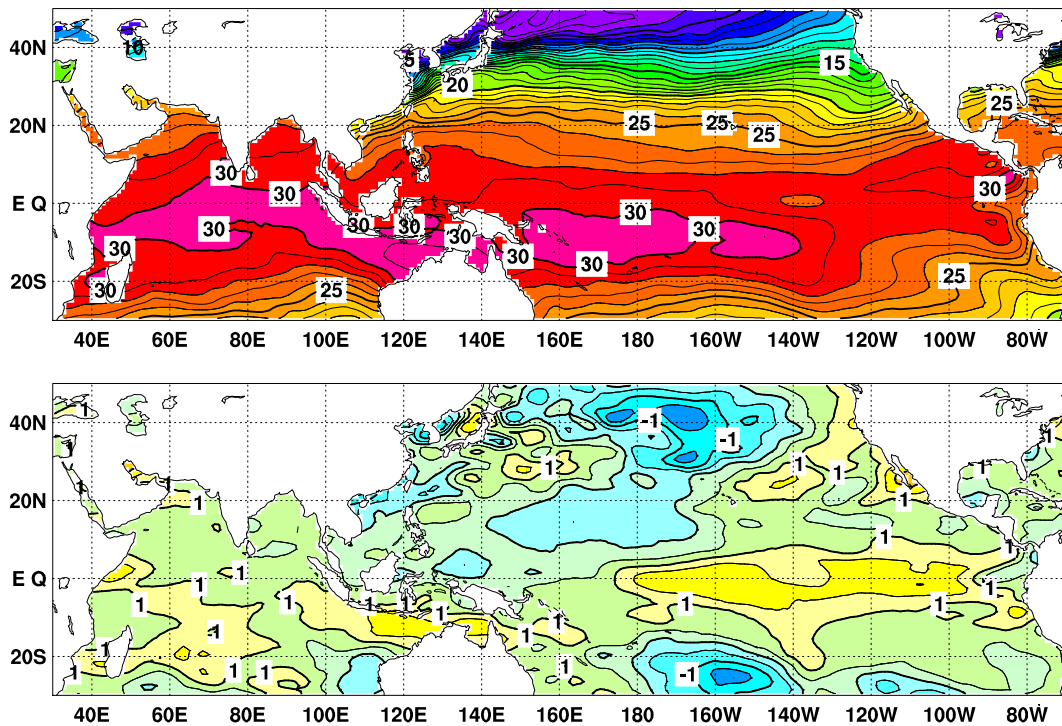
図2 2016年3月の海面水温図（上）及び平年偏差図（下）
