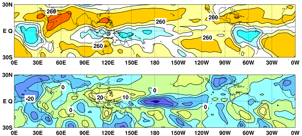
図6 外向き長波放射量 (OLR) (上) 及び年偏差 (下) の分布図 (2016年3月)
