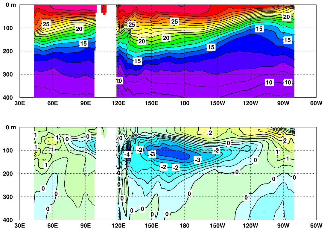
図3 2016年3月のインド洋から太平洋の赤道に沿った水温（上）及び平年偏差（下）の断面図
