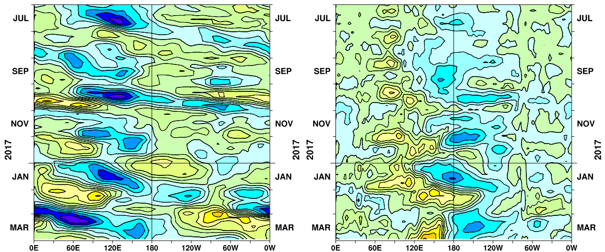
図10 赤道付近における対流圏上層 (200hPa) の速度ポテンシャルの平年偏差 (a) 及び対流圏下層 (850hPa) の東西風速の平年偏差 (b) の経度-時間断面図
