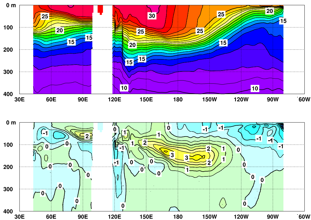
図5 2018年3月のインド洋から太平洋の赤道に沿った水温（上）及び平年偏差（下）の断面図
