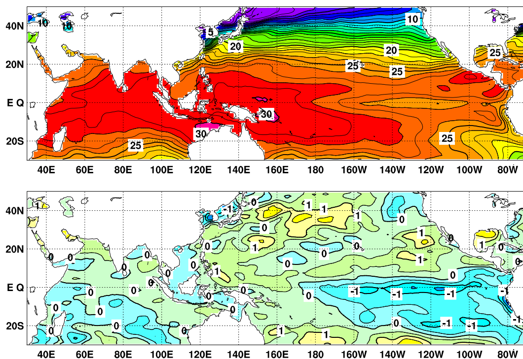
図4 2018年3月の海面水温図（上）及び平年偏差図（下）
