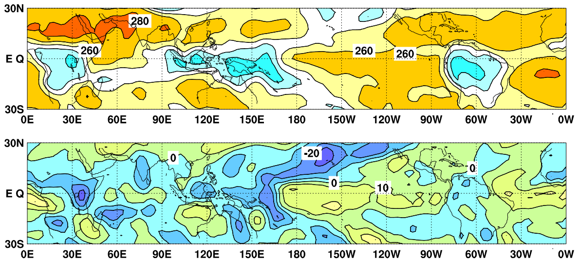
図9 外向き長波放射量 (OLR) (上) 及び平年偏差 (下) の分布図 (2018年3月)
