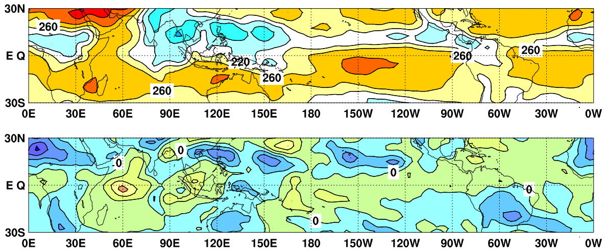
図9 外向き長波放射量 (OLR) (上) 及び平年偏差 (下) の分布図 (2018年8月)
