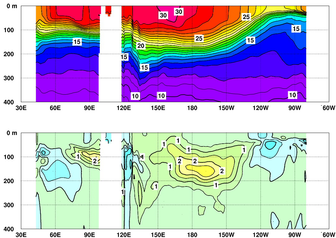
図5 2018年8月のインド洋から太平洋の赤道に沿った水温(上)及び平年偏差(下)の断面図
