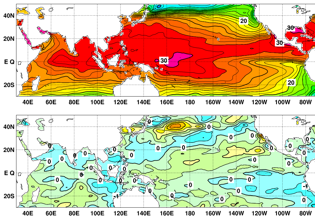
図4 2018年8月の海面水温図(上)及び平年偏差図(下)
