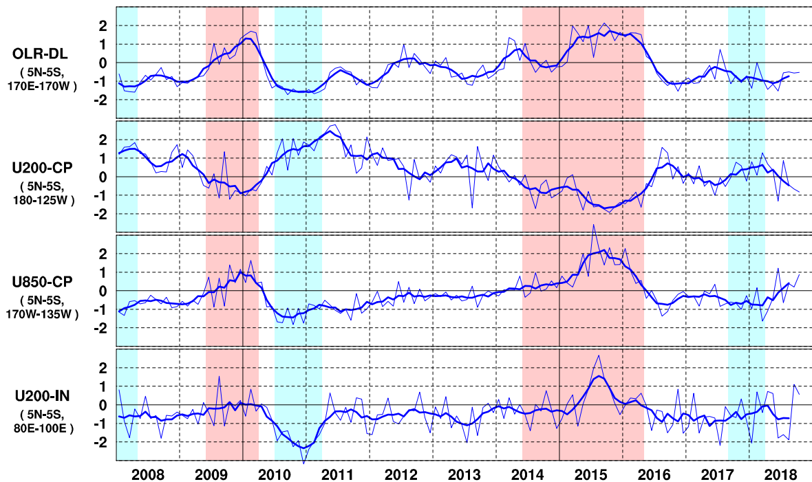
図8 日付変更線付近のOLR指数(OLR-DL)、対流圏上層(200hPa)の赤道東西風指数(U200-CP)、対流圏下層(850hPa)の赤道東西風指数(U850-CP)、インド洋における対流圏上層(200hPa)の赤道東西風指数(U200-IN)の時系列(上から順に) 折線は月平均値、滑らかな太線は5か月移動平均値を示す(平年値は1981~2010年の30年平均値)。赤色の陰影はエルニーニョ現象の発生期間を、青色の陰影はラニーニャ現象の発生期間を示している。
