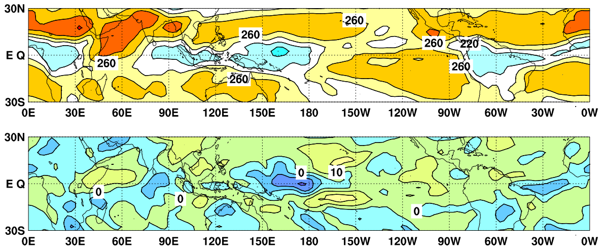
図9 外向き長波放射量 (OLR) (上) 及び平年偏差 (下) の分布図 (2019年4月)
