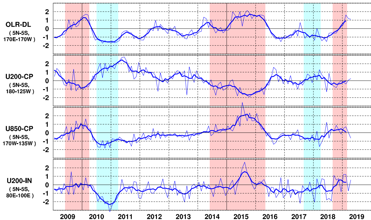
図 8 日付変更線付近の OLR 指数 (OLR-DL)、対流圏上層 (200hPa) の赤道東西風指数 (U200-CP)、対 流圏下層 (850hPa) の赤道東西風指数 (U850-CP)、インド洋における対流圏上層 (200hPa) の赤道東西風指数 (U200-IN) の時系列 (上から順に) 折線は月平均値、滑らかな太線は 5 か月移動平均値を示す (平年値は 1981~2010 年の 30 年平均値)。赤色の陰影はエル ニニョ現象の発生期間を、青色の陰影はラニーニャ現象の発生期間を示している。
