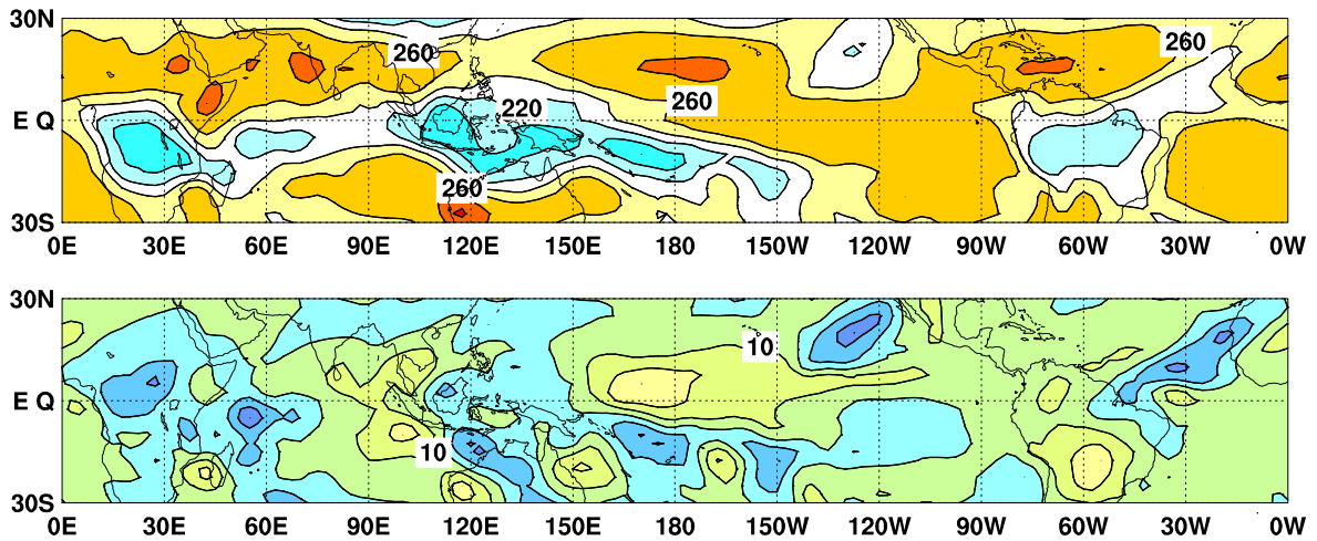
図9 外向き長波放射量 (OLR) (上) 及び平年偏差 (下) の分布図 (2022年1月)
