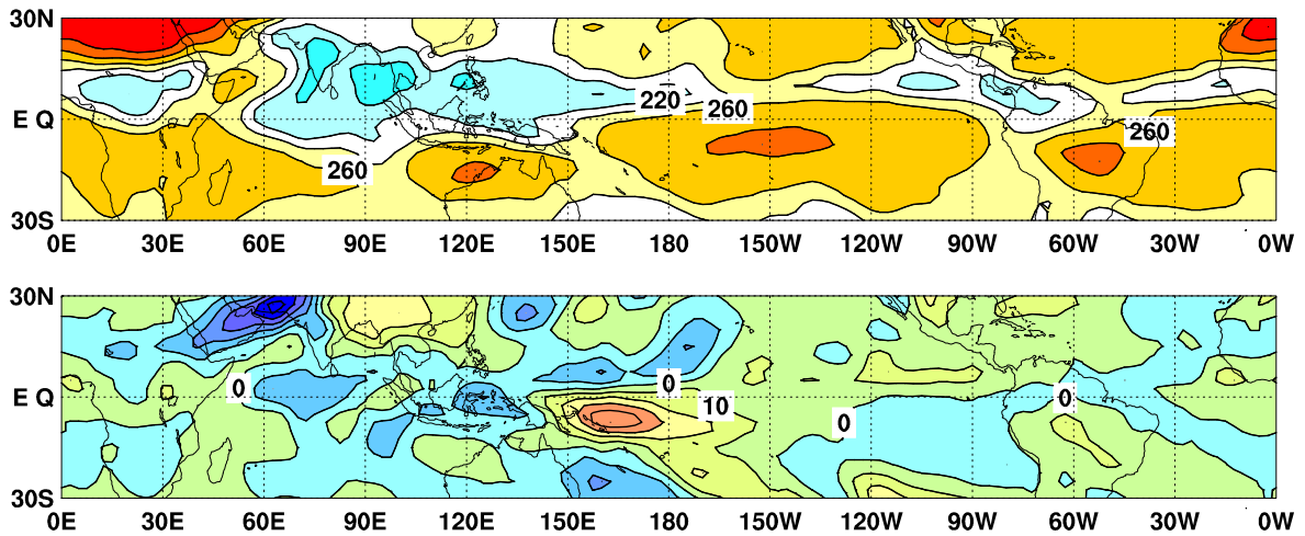
図9 外向き長波放射量 (OLR) (上) 及び年偏差 (下) の分布図 (2022年7月)
