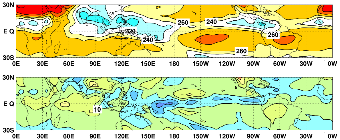
図9 外向き長波放射量 (OLR) (上) 及び年偏差 (下) の分布図 (2023年7月)
