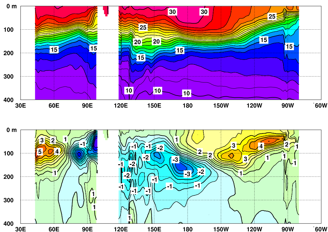
図5 2023年12月のインド洋から太平洋の赤道に沿った水温（上）及び平年偏差（下）の断面図
