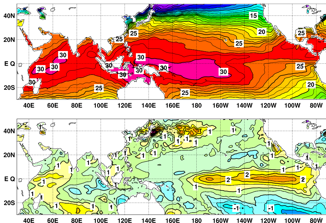
図4 2023年12月の海面水温図（上）及び平年偏差図（下）
