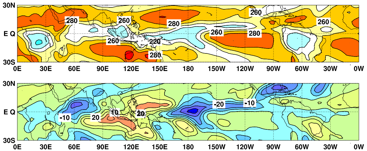
図9 外向き長波放射量 (OLR) (上) 及び年偏差 (下) の分布図 (2023年12月)
