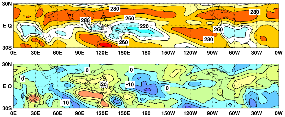
図9 外向き長波放射量 (OLR) (上) 及び平年偏差 (下) の分布図 (2024年2月)
