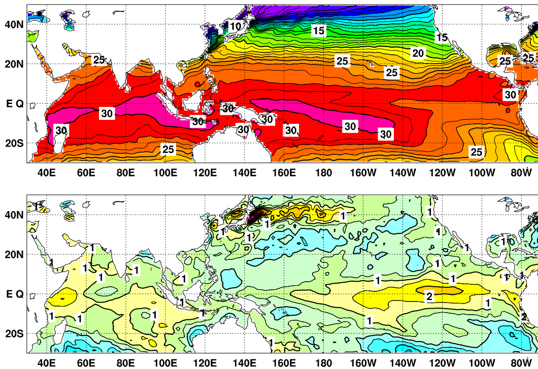
図4 2024年2月の海面水温図(上)及び平年偏差図(下)
