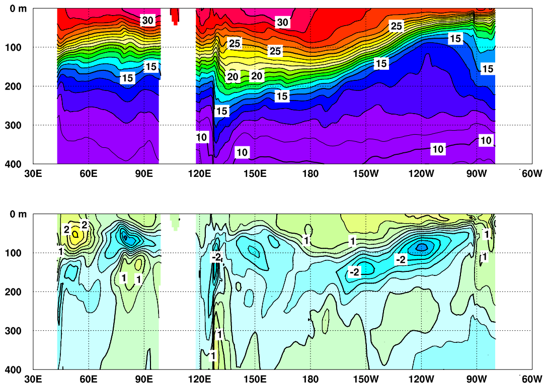
図5 2024年2月のインド洋から太平洋の赤道に沿った水温(上)及び平年偏差(下)の断面図
