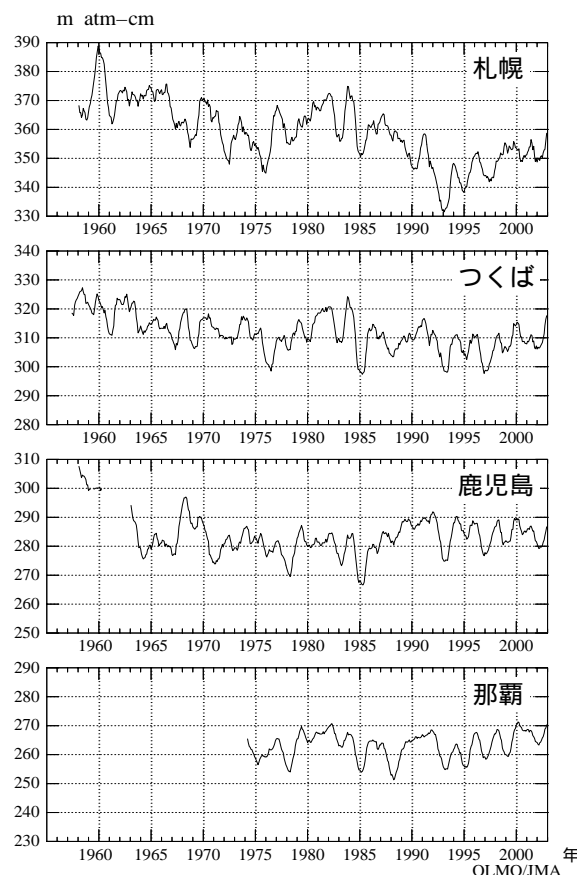
図3-1-2: 季節変動除去後のオゾン全量の推移 図3-1-1のデータから季節変動を除去した後13カ月移動平均をした。
