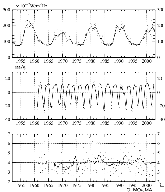
図3 - 1 - 3 : オゾン変動に影響する既知の自然要因
