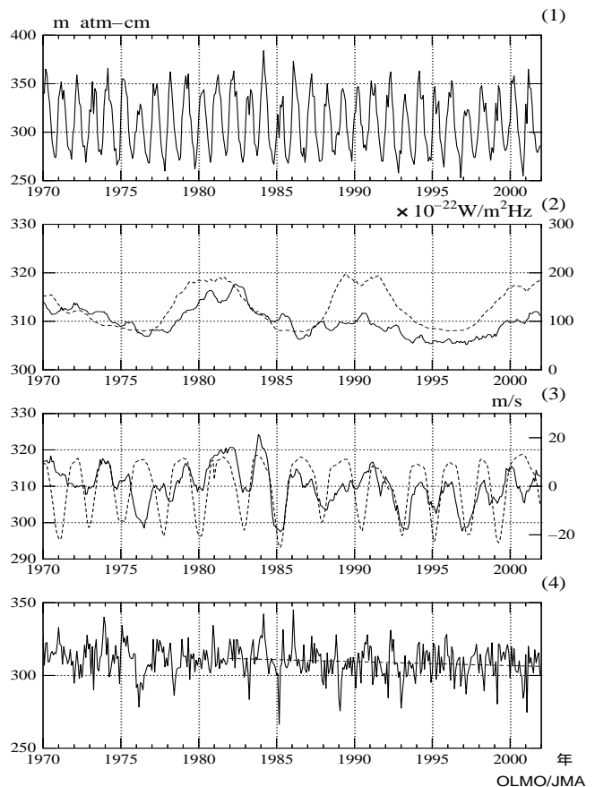
図3 - 1 - 4 : つくばにおけるオゾン全量のトレンド解析例
