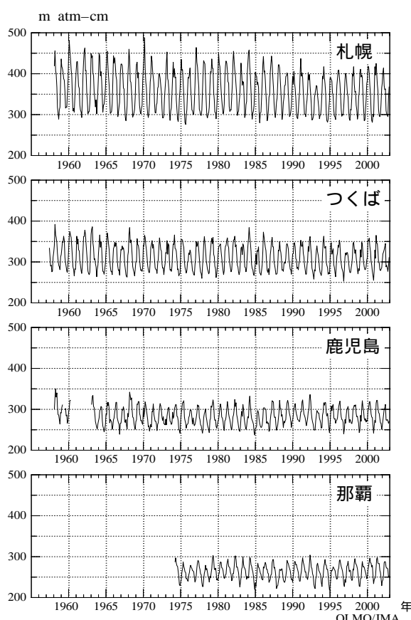
図3-1-1: 日本上空のオゾン全量の月平均値 札幌、つくば、鹿児島、那覇についての観測開始から2002年12月までのオゾン全量の月平均値。
