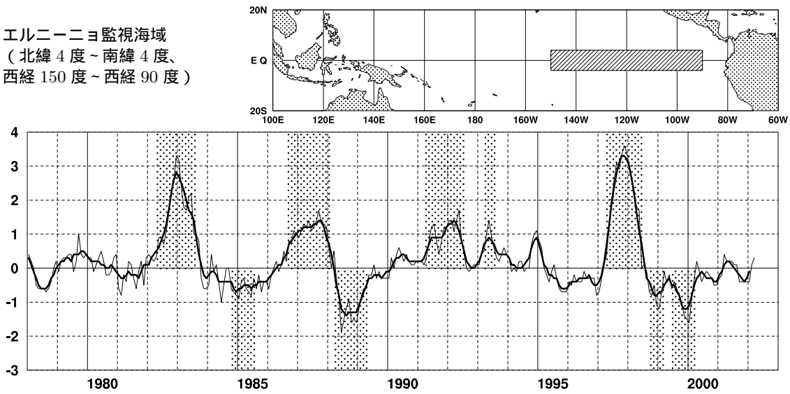
図 1 エルニーニョ監視海域の月平均海面水温の基準値との差 (°C) の推移 (1978 年 1 月 ~ 2002 年 3 月)。折線は月平均値、滑らかな太線は 5 か月移動平均値を示し、正の値は基準値より高いことを示す。エルニーニョ現象の発生期間は上側に、ラニーニャ現象の発生期間は下側に、それぞれ陰影を施してある (基準値は 1961 ~ 1990 年の 30 年平均値)。
