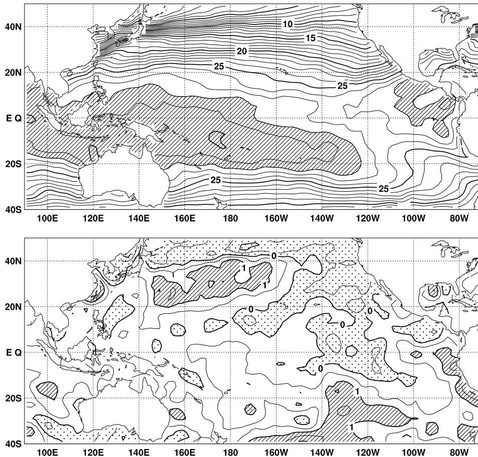
図 2 2002 年 3 月の海面水温図 (上) 及び平年偏差図 (下)。海面水温図の大線は 5°C 毎、細線は 1°C 毎の、平年偏差図の大線は 1°C 毎、細線は 0.5°C 毎の等値線を示す。海面水温図の陰影部は 28°C 以上の領域を、偏差図の濃い (薄い) 陰影部は +1°C 以上の正偏差域 (0°C 以下の負偏差域) を示す (平年値は 1971 ~ 2000 年の 30 年平均値)。
