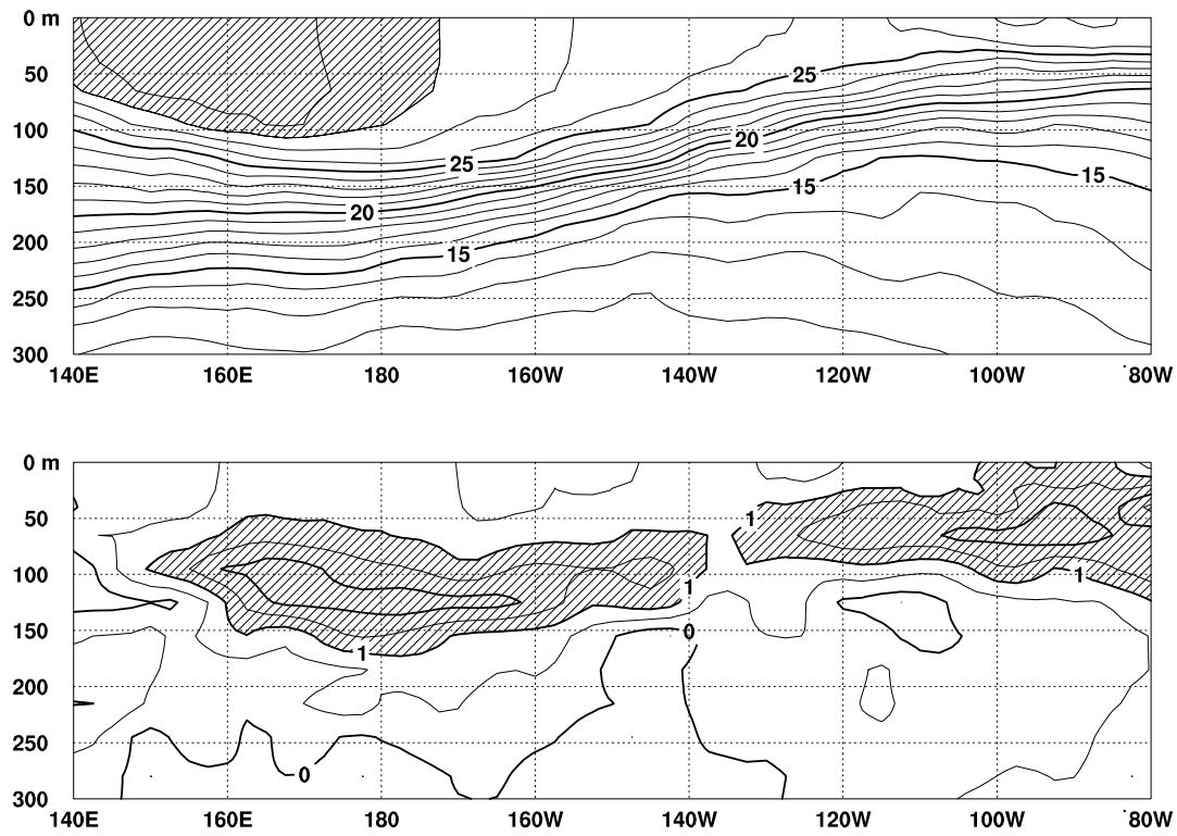
図3 2002年3月の太平洋の赤道に沿った水温(上)及び平年偏差(下)の断面図(海洋データ同化システムによる)。上図の等値線間隔は 1^{\circ}\text{C} で 28^{\circ}\text{C} 以上には陰影を施し、下図の等値線間隔は 0.5^{\circ}\text{C} で +1^{\circ}\text{C} 以上( -1^{\circ}\text{C} 以下)の偏差には濃い(薄い)陰影を施した(平年値は1987~2000年の14年平均値)。
