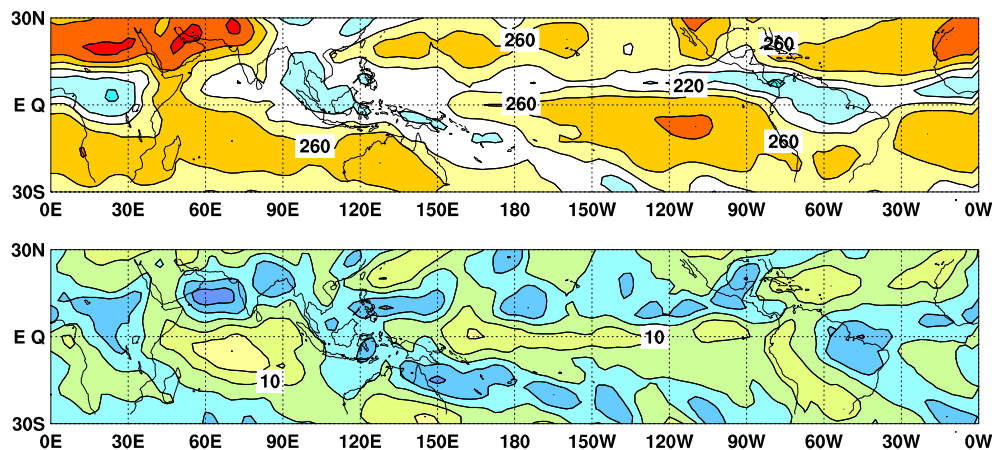
図 6 2006 年 5 月の外向き長波放射量 (OLR) ( 上 ) 及び平年偏差 ( 下 ) の分布図。OLR の値が小さいほど、対流活動が活発であることを示す。上図は 20\text{W/m}^2 毎、下図は 10\text{W/m}^2 毎に等値線を描いている ( 平年値は 1979 ~ 2000 年の 22 年平均値 )。OLR データは米国海洋大気庁 ( NOAA ) から提供されたものである。
