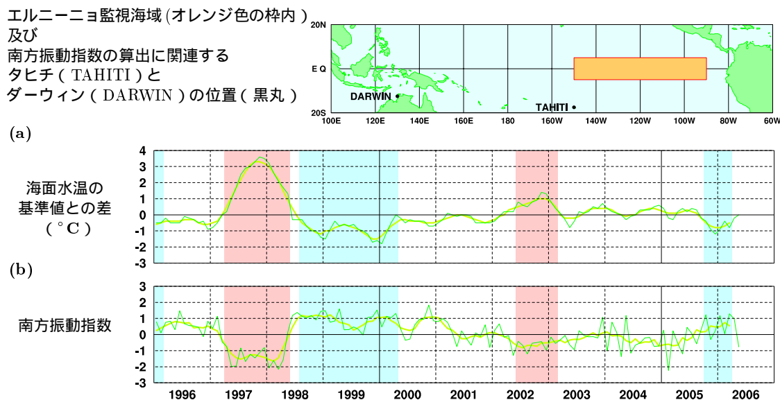
図1 エルニーニョ監視海域の海面水温の基準値との差( ^{\circ}\text{C} )(a)と南方振動指数(b)の推移(1996年1月~2006年5月)。折線は月平均値、滑らかな太線は5か月移動平均値を示す(海面水温の基準値はその年の前年までの30年間の各月の平均値、南方振動指数の平年値は1971~2000年の30年平均値)。赤色の陰影はエルニーニョ現象の発生期間を、青色の陰影はラニーニャ現象の発生期間を示している。
