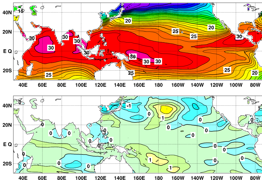
図 2 2006 年 5 月の海面水温図 ( 上 ) 及び平年偏差図 ( 下 )。海面水温図の太線は 5^{\circ}\text{C} 毎、細線は 1^{\circ}\text{C} 毎の、平年偏差図の太線は 1^{\circ}\text{C} 毎、細線は 0.5^{\circ}\text{C} 毎の等値線を示す ( 平年値は 1971 ~ 2000 年の 30 年平均値 )。
