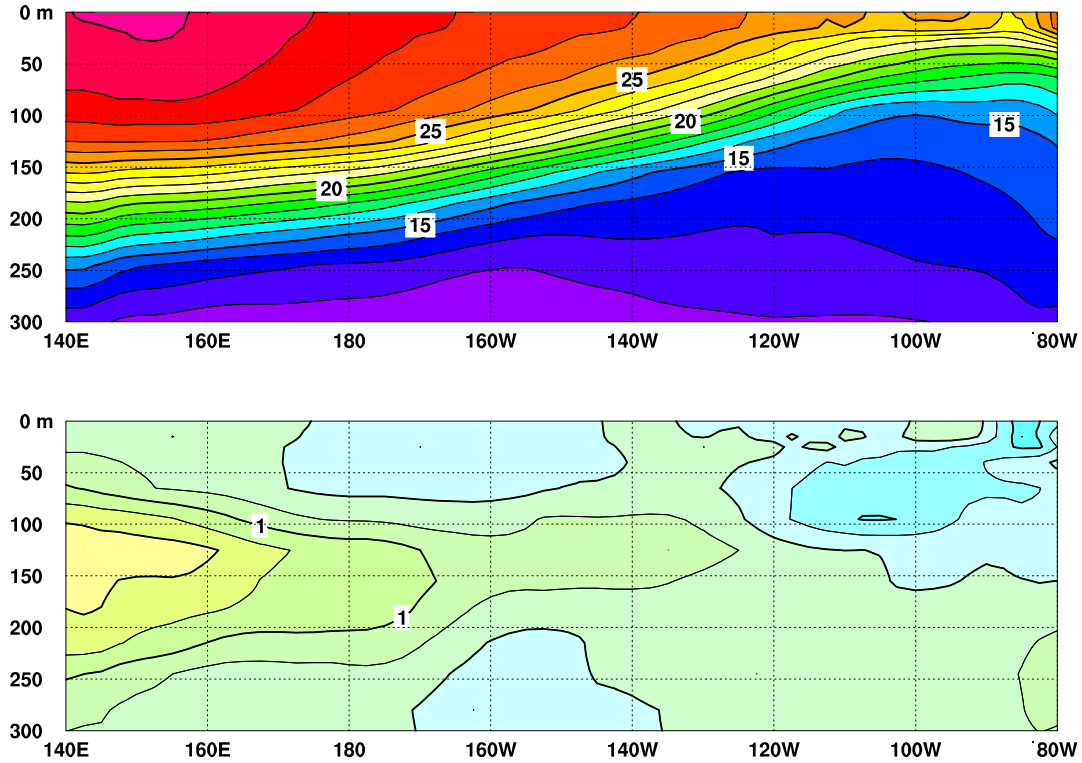
図3 2006年5月の太平洋の赤道に沿った水温(上)及び平年偏差(下)の断面図(海洋データ同化システムによる)。上図の等値線間隔は 1^{\circ}\text{C} 、下図の等値線間隔は 0.5^{\circ}\text{C} (平年値は1987~2005年の19年平均値)。
