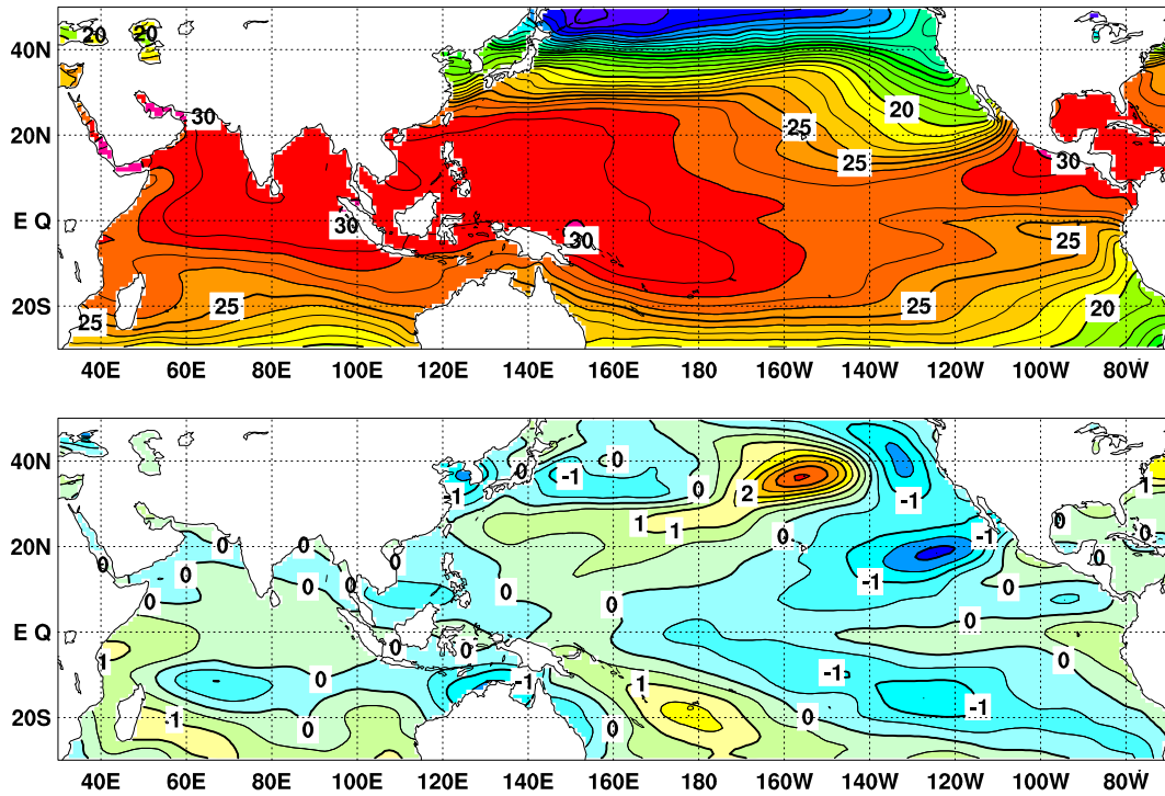
図 2 2011 年 6 月の海面水温図 ( 上 ) 及び 年 間 偏 差 図 ( 下 )
