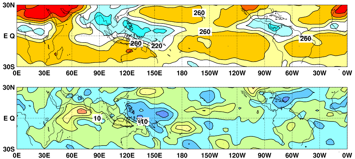
図6 外向き長波放射量 (OLR) (上) 及び年偏差 (下) の分布図 (2011 年 6 月)
