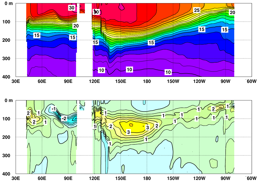
図 3 2011 年 6 月のインド 洋 から 太 平 洋 の 赤 道 に 沿 っ た 水 温 ( 上 ) 及 び 年 間 偏 差 ( 下 ) の 断 面 図
