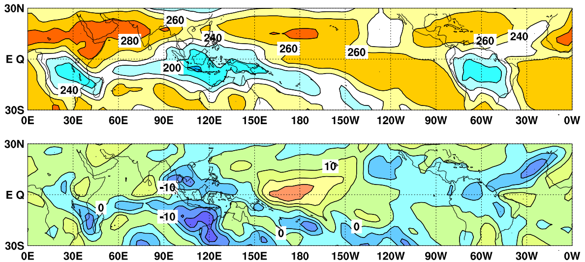
図6 外向き長波放射量 (OLR) (上) 及び年偏差 (下) の分布図 (2012 年 1 月)
