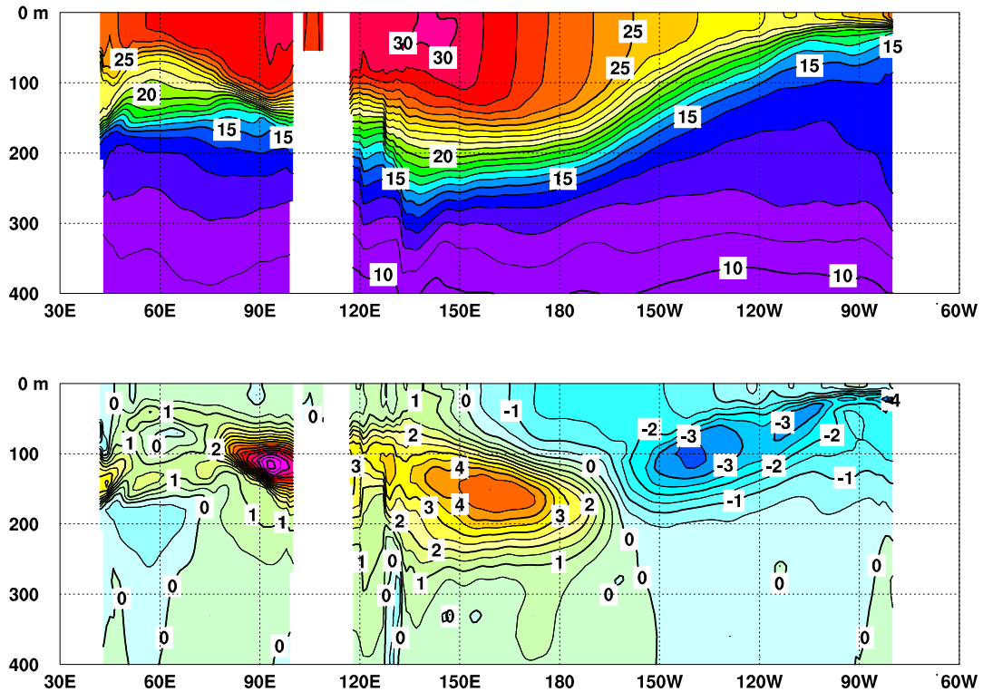
図 3 2012 年 1 月のインド洋から太平洋の赤道に沿った水温 ( 上 ) 及び平年偏差 ( 下 ) の断面図
