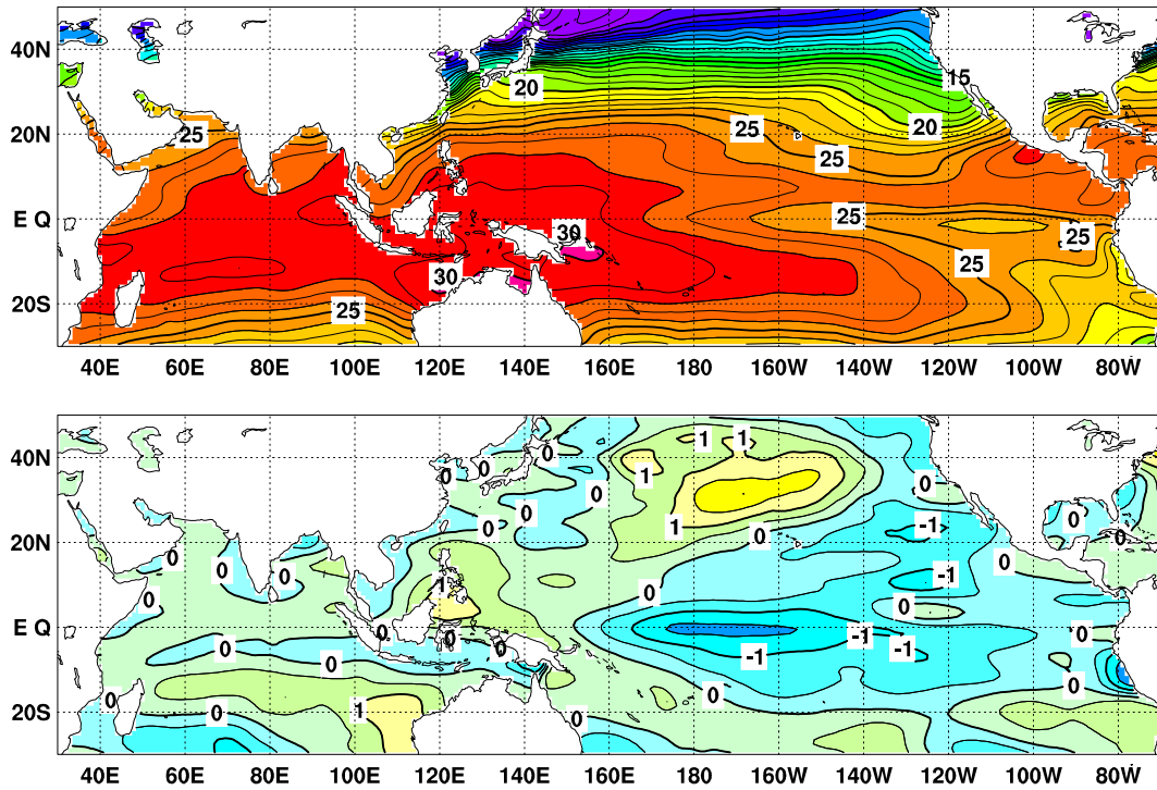
図 2 2012 年 1 月の海面水温図 ( 上 ) 及び平年偏差図 ( 下 )
