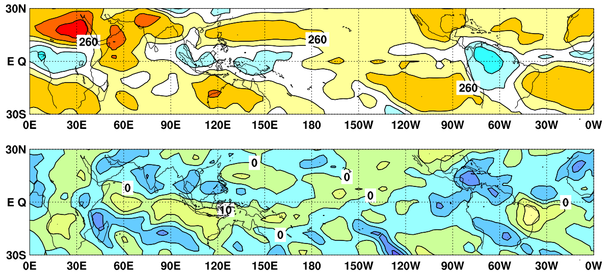
図6 外向き長波放射量 (OLR) (上) 及び年偏差 (下) の分布図 (2012 年 4 月)
