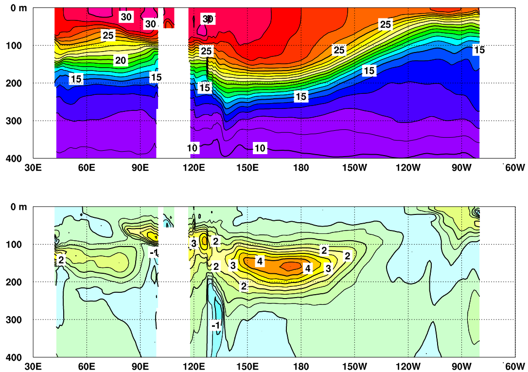
図 3 2012 年 4 月のインド洋から太平洋の赤道に沿った水温 ( 上 ) 及び平年偏差 ( 下 ) の断面図
