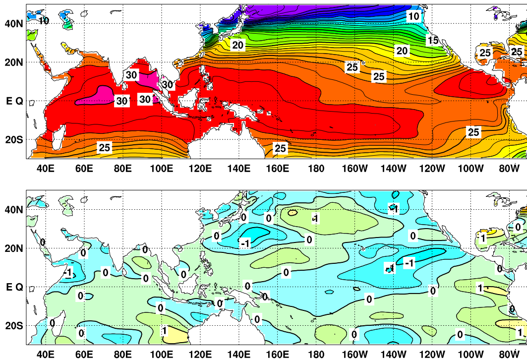
図 2 2012 年 4 月の海面水温図 ( 上 ) 及び平年偏差図 ( 下 )
