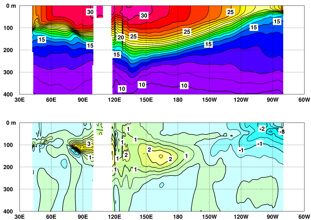
図 3 2013 年 6 月のインド洋から太平洋の赤道に沿った水温 ( 上 ) 及び平年偏差 ( 下 ) の断面図
