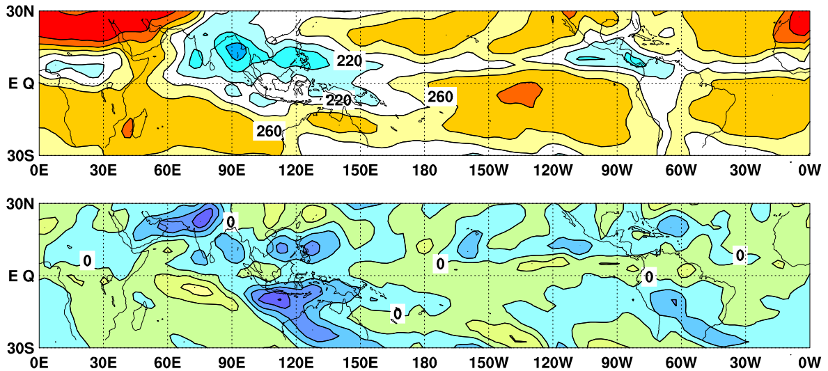
図6 外向き長波放射量 (OLR) (上) 及び年偏差 (下) の分布図 (2013 年 6 月)
