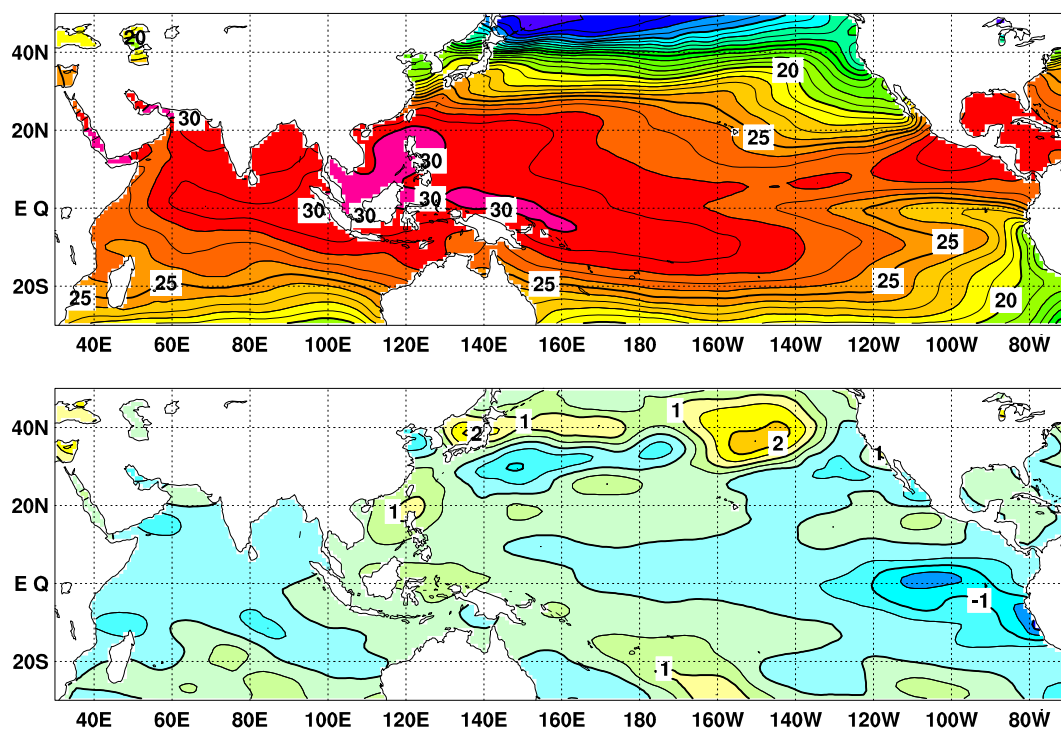
図 2 2013 年 6 月の海面水温図 ( 上 ) 及び平年偏差図 ( 下 )
