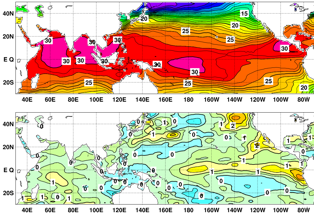
図2 2015年5月の海面水温図(上)及び平年偏差図(下)
