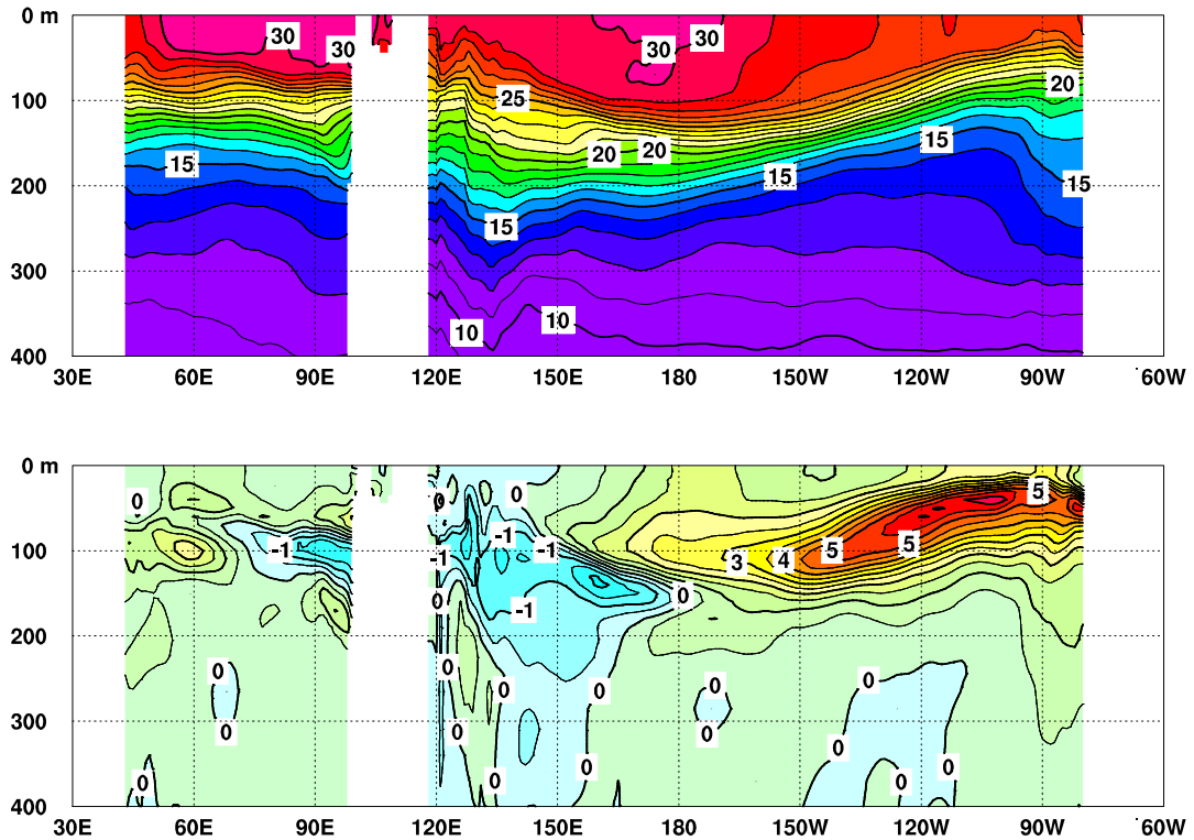
図3 2015年5月のインド洋から太平洋の赤道に沿った水温(上)及び平年偏差(下)の断面図
