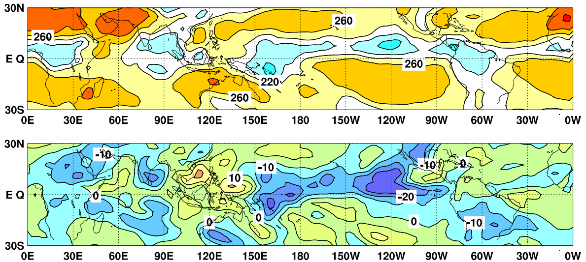
図6 外向き長波放射量 (OLR) (上) 及び年偏差 (下) の分布図 (2015 年 5 月)
