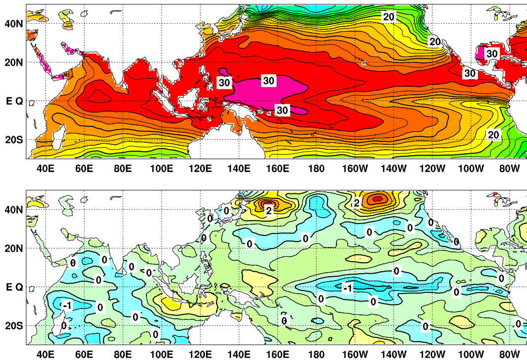
図4 2016年9月の海面水温図（上）及び平年偏差図（下）
