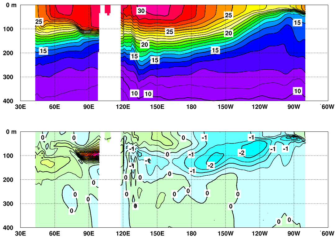
図5 2016年9月のインド洋から太平洋の赤道に沿った水温（上）及び平年偏差（下）の断面図
