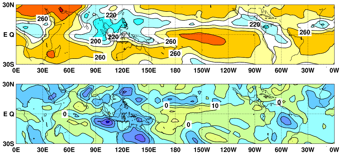
図 8 外向き長波放射量 (OLR) (上) 及び年偏差 (下) の分布図 (2016 年 9 月)
