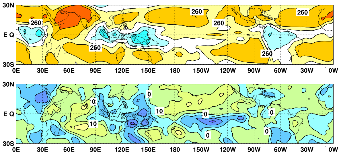
図8 外向き長波放射量 (OLR) (上) 及び年偏差 (下) の分布図 (2017年4月)
