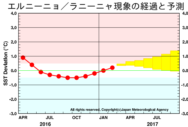
図 1 エルニーニョ監視海域の海面水温の基準値との差の 5 か月移動平均値 2 月までの経過（観測値）を折れ線グラフで、エルニーニョ予測モデルによる予測結果（70%の確率で入ると予想される範囲）をボックスで示している。指数が赤／青の範囲に入っている期間がエルニーニョ／ラニーニャ現象の発生期間である。
