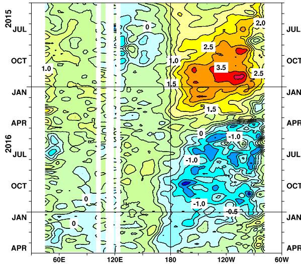
図6 インド洋から太平洋の赤道に沿った海面水温 年偏差の経度-時間断面図 太線は1°C毎、細線は0.5°C毎の等値線を示す（平 年値は1981~2010年の30年平均値）。図中白く抜け ている部分は陸地である。
