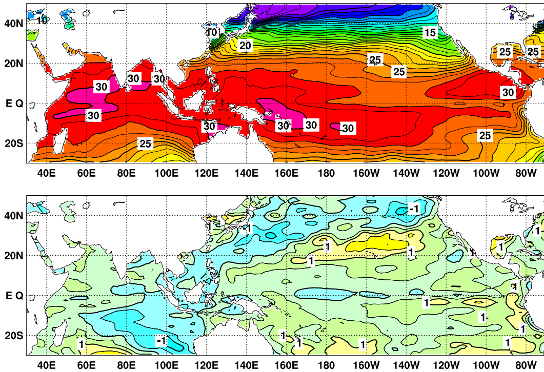
図4 2017年4月の海面水温図（上）及び平年偏差図（下）
