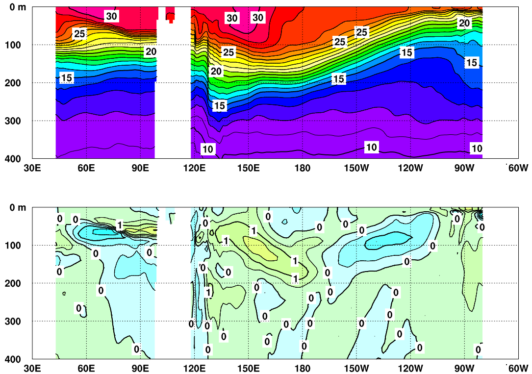
図5 2017年4月のインド洋から太平洋の赤道に沿った水温（上）及び平年偏差（下）の断面図
