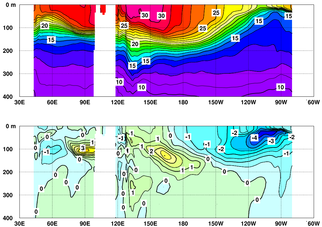
図5 2017年12月のインド洋から太平洋の赤道に沿った水温（上）及び平年偏差（下）の断面図
