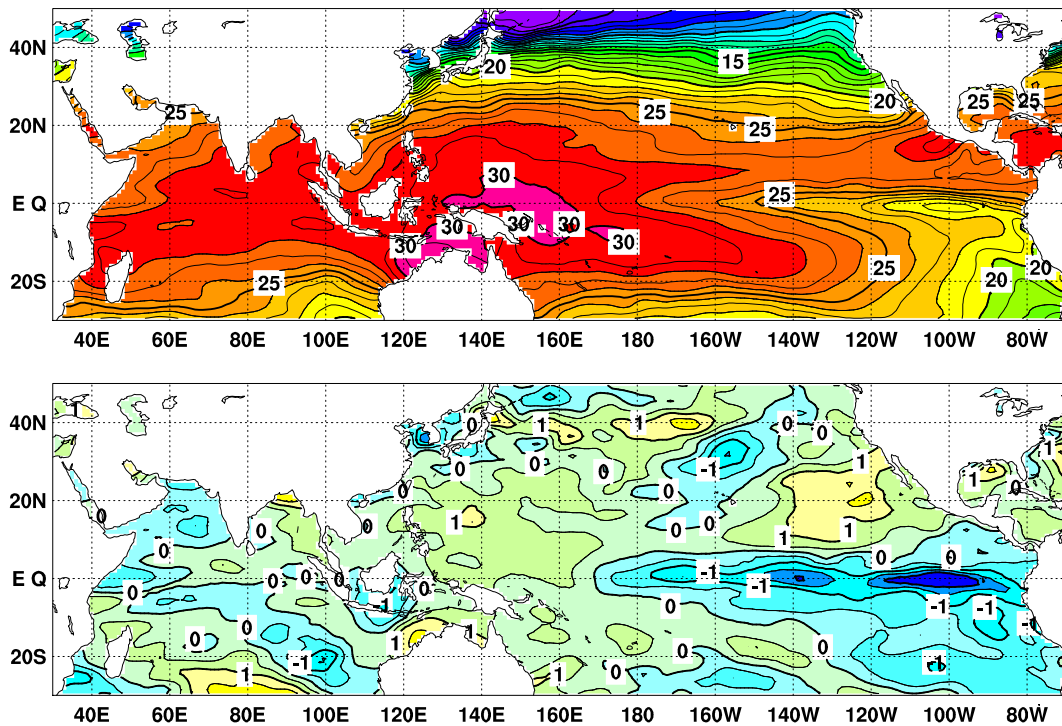
図4 2017年12月の海面水温図（上）及び平年偏差図（下）
