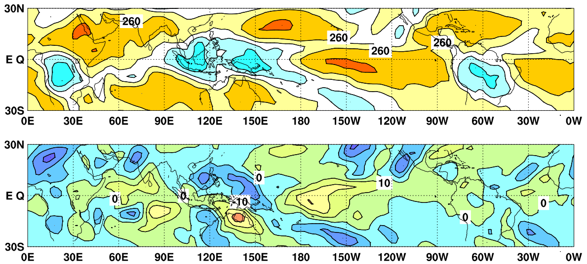
図9 外向き長波放射量 (OLR) (上) 及び平年偏差 (下) の分布図 (2017年12月)
