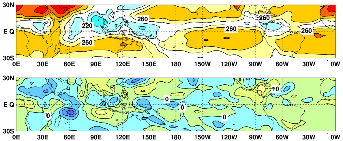
図9 外向き長波放射量 (OLR) (上) 及び平年偏差 (下) の分布図 (2019年6月)
